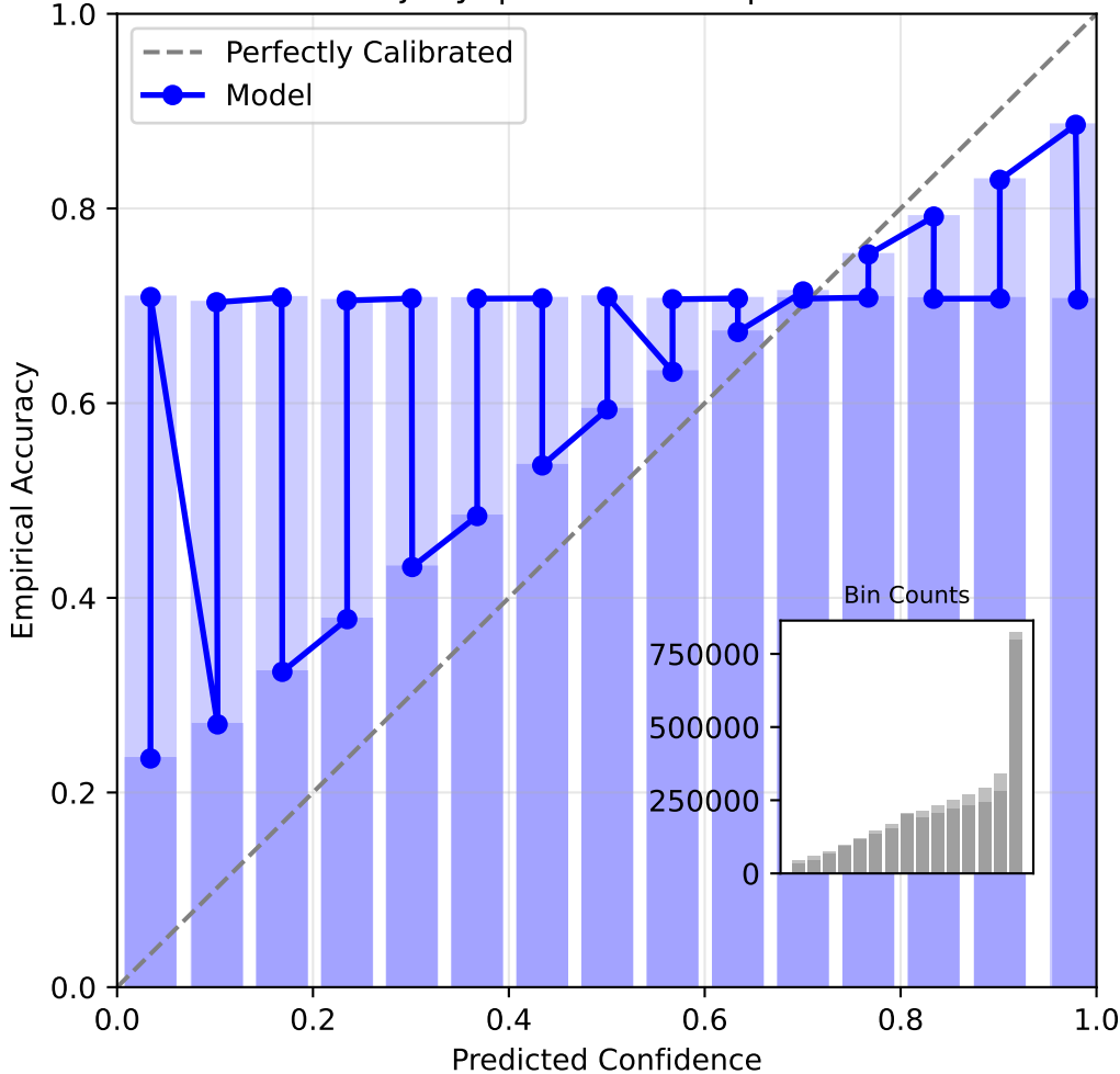
Reliability Diagram: simplekt (dense) Dataset: junyi | ECE: 0.2267 | N: 3072767
