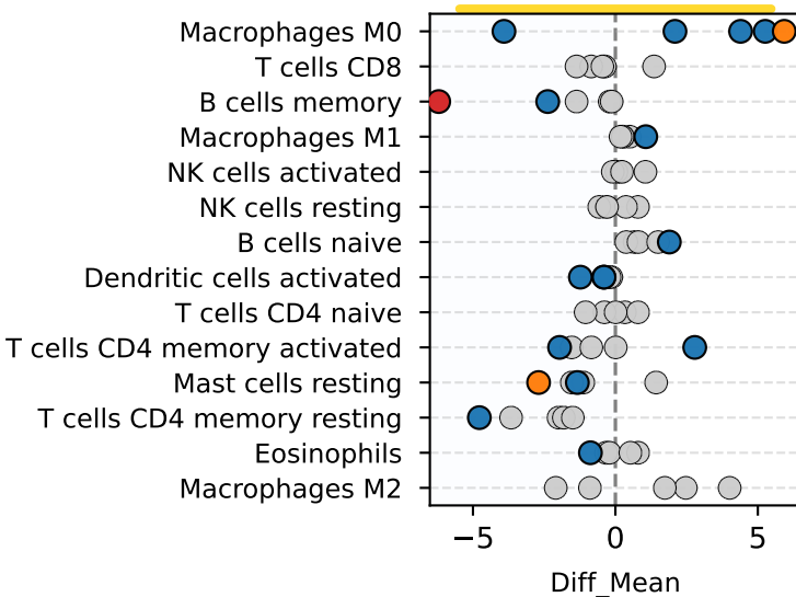
TVAE
