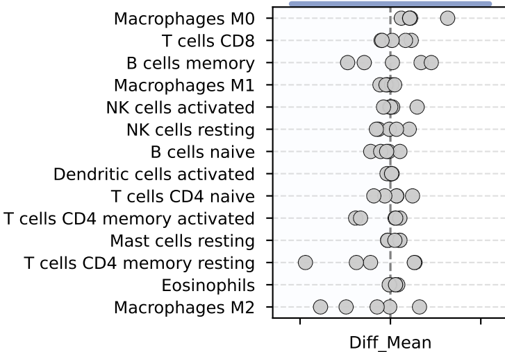
TVAE
