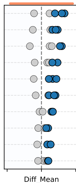
TVAE
