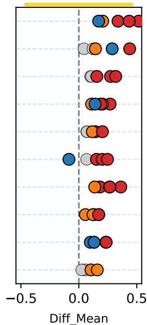
TVAE
