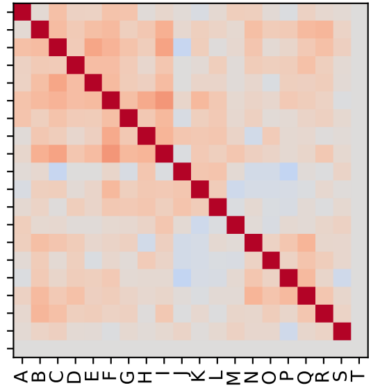
TVAE
