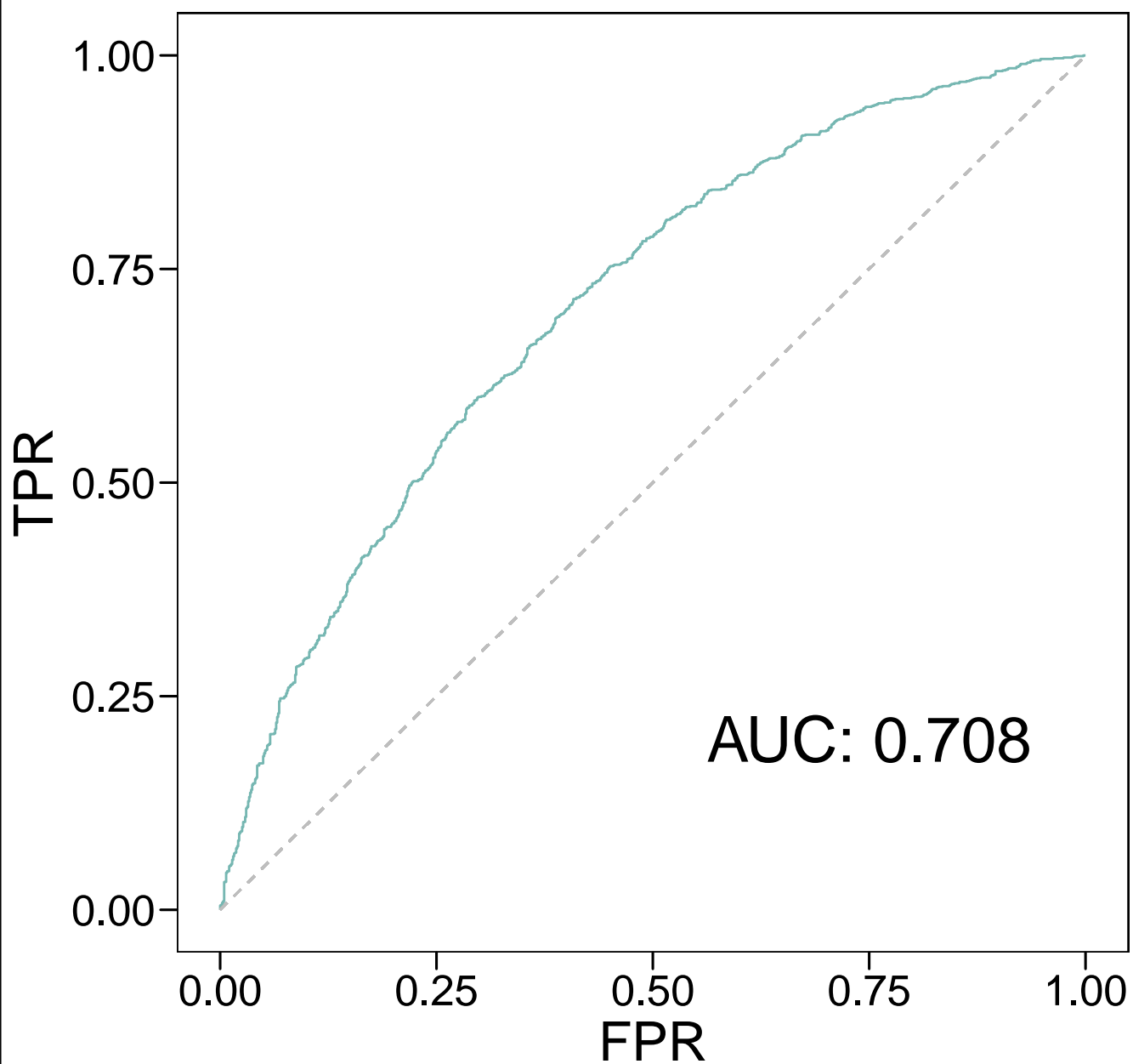
rop_any ROC
