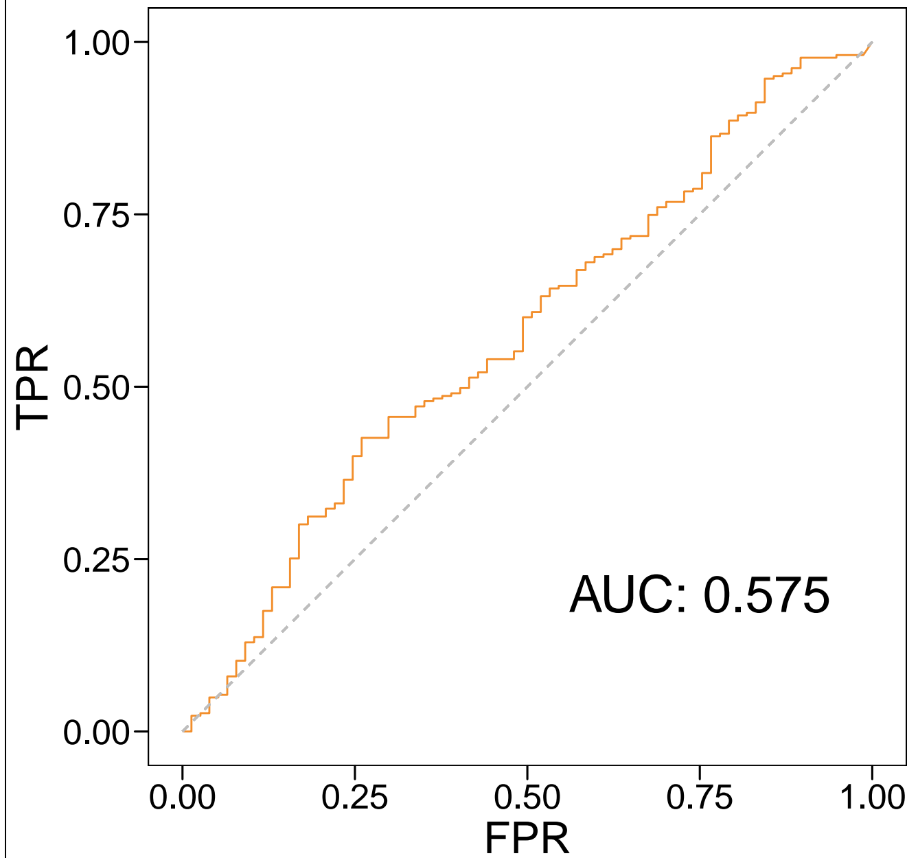
ivh_any ROC
