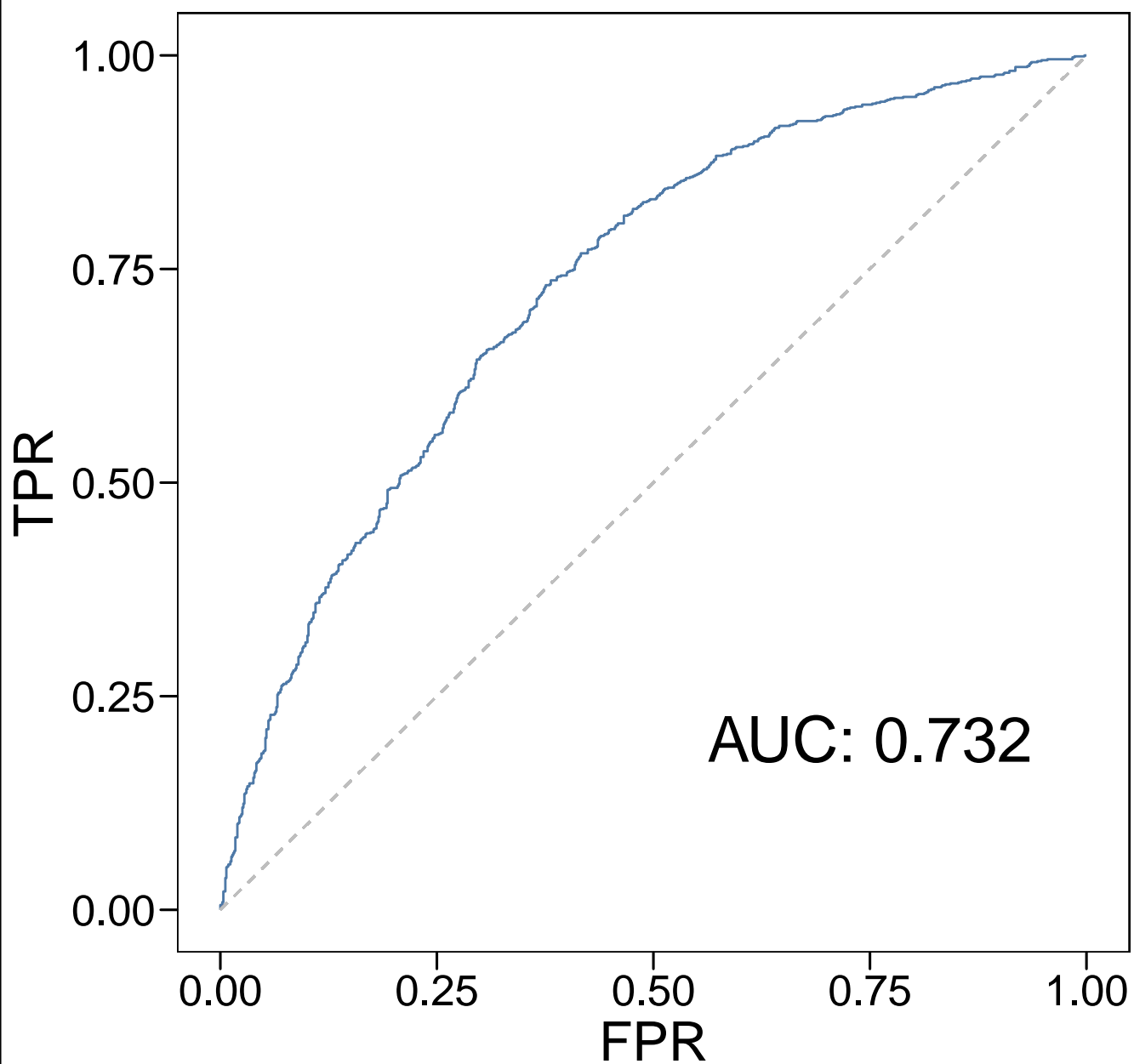
bpd_any ROC
