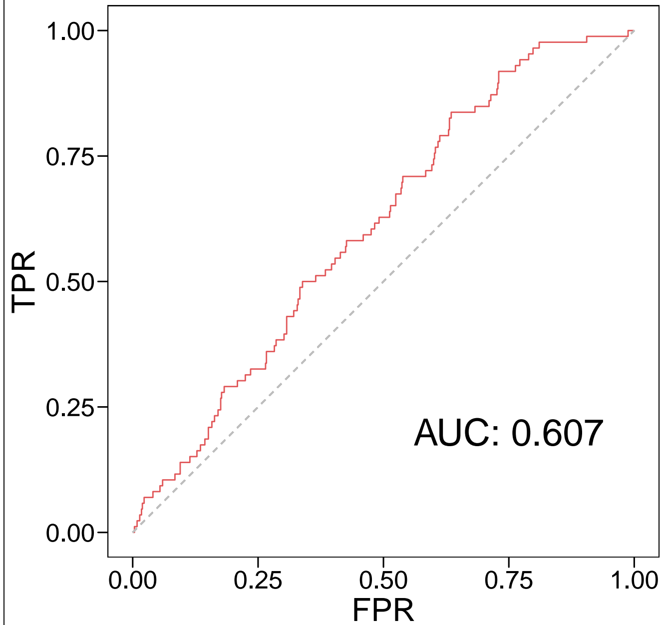
nec_any ROC
