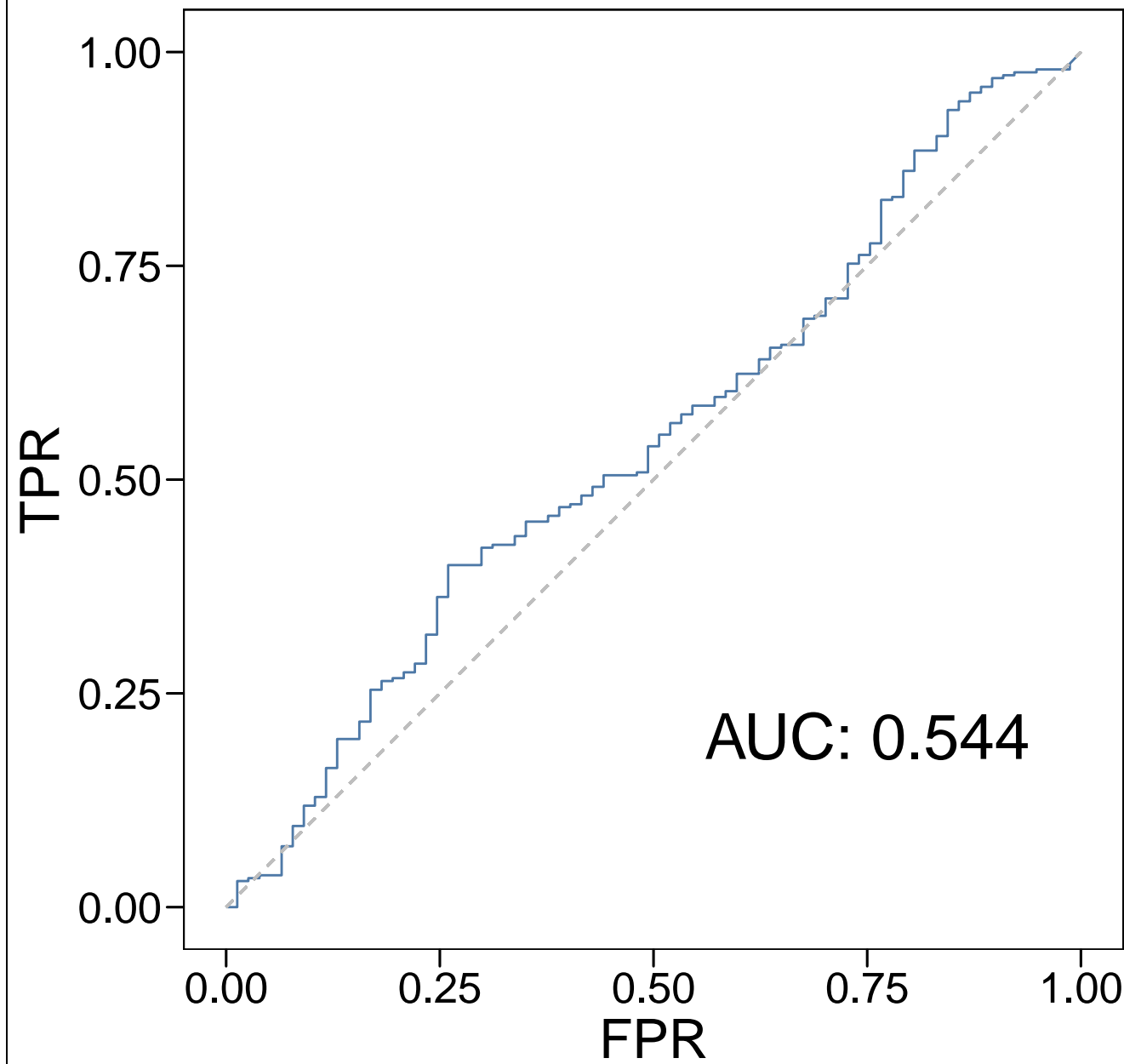
bpd_any ROC
