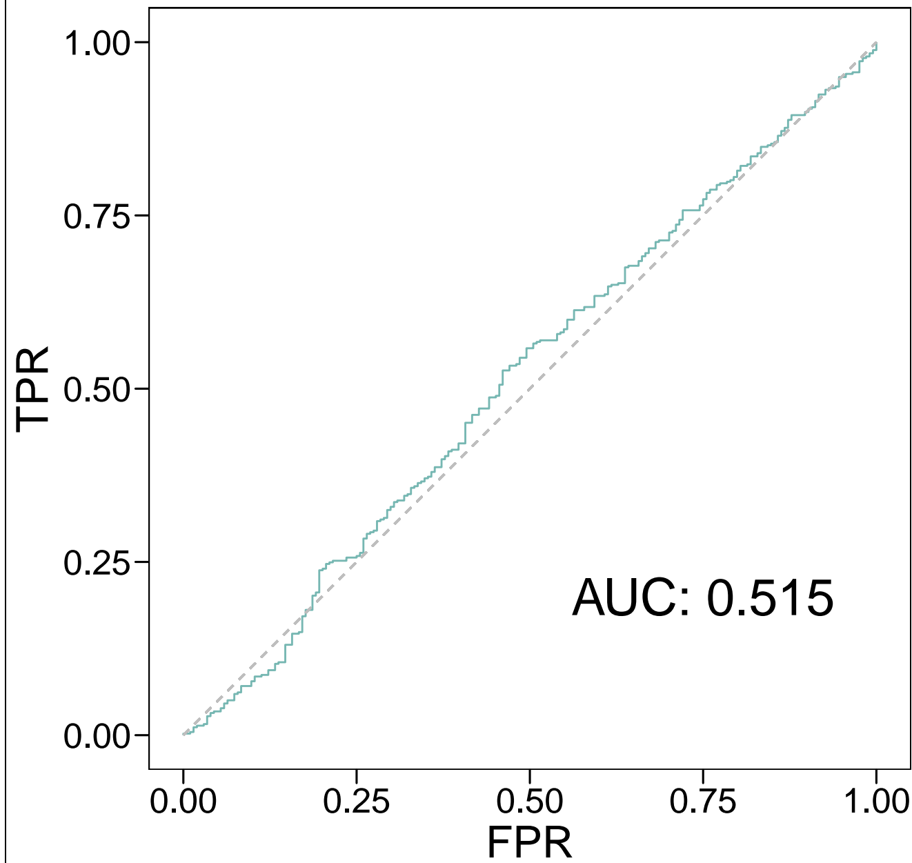
rop_any ROC
