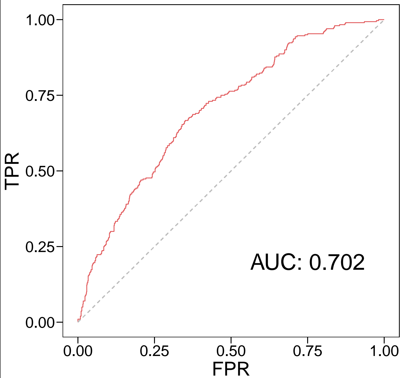
nec_any ROC
