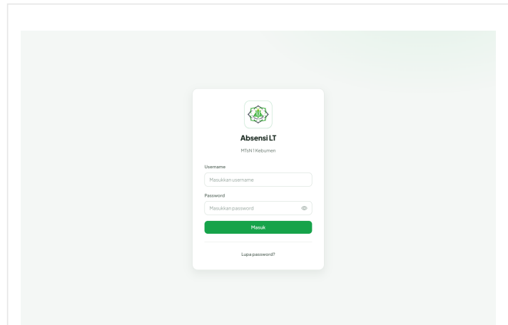
Halaman login
