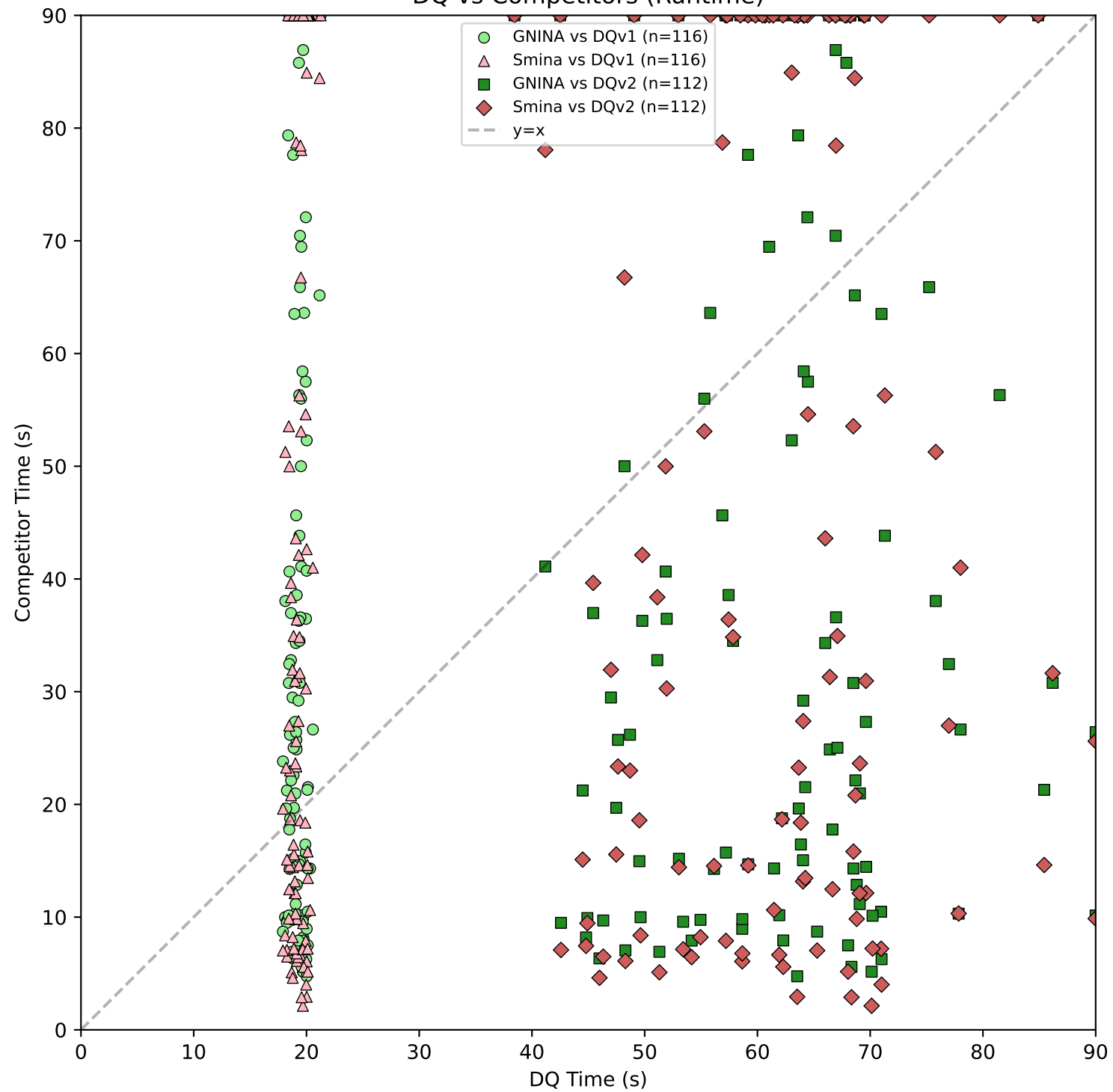
DQ vs Competitors (Runtime)
