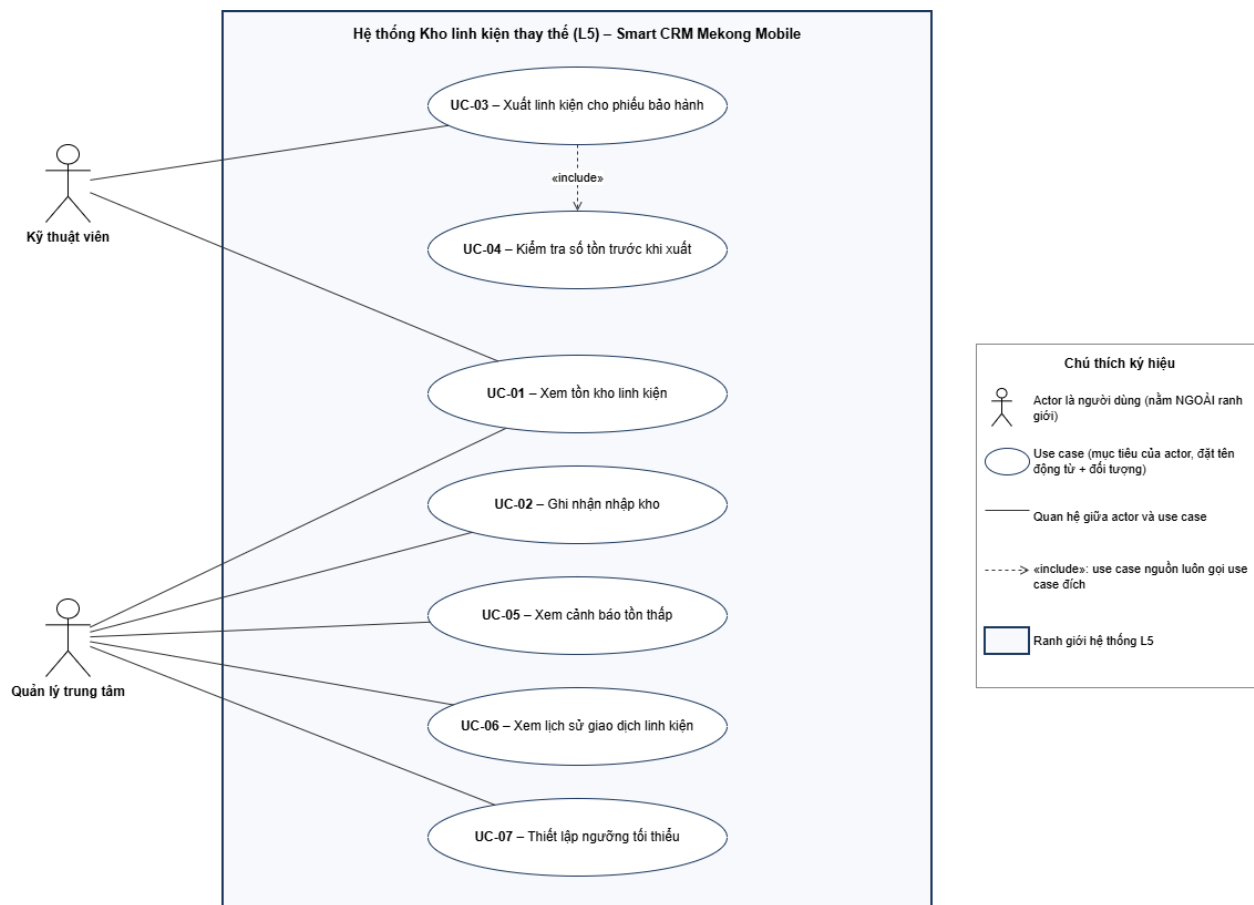
Hình 2.1: Sơ đồ Use Case Diagram – Luồng L5: Kho linh kiện thay thế (docs/usecase.drawio)
