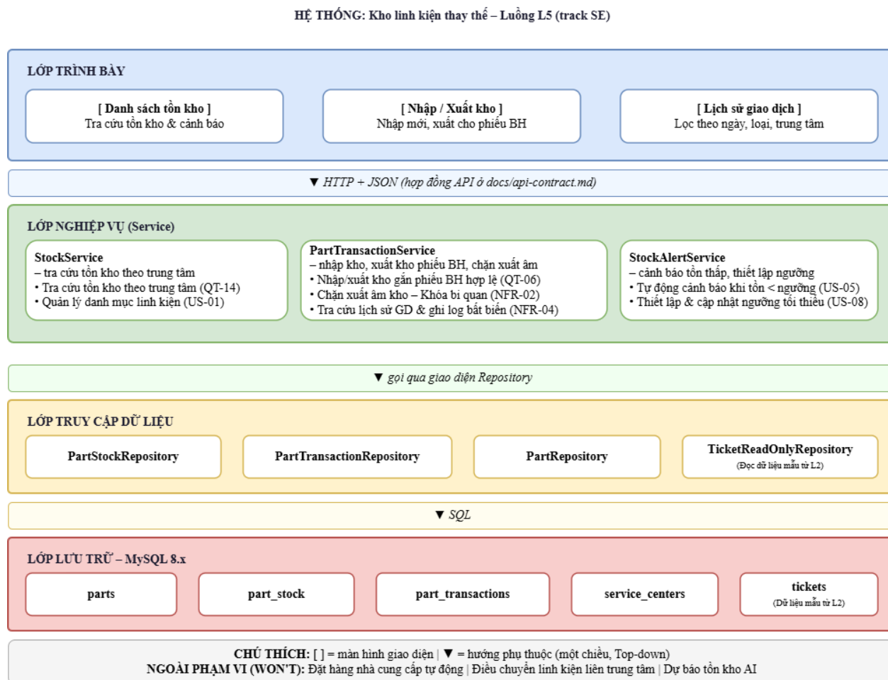
Hình 3.1: Sơ đồ Kiến trúc Phân tầng 4 lớp – Luồng L5: Kho linh kiện thay thế (docs/architecture.drawio)
