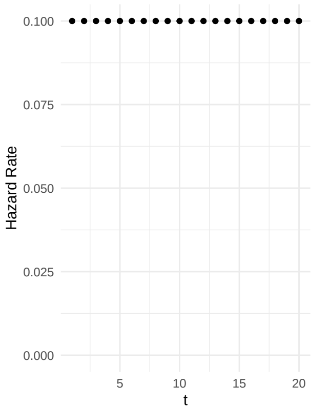
Hazard Function
