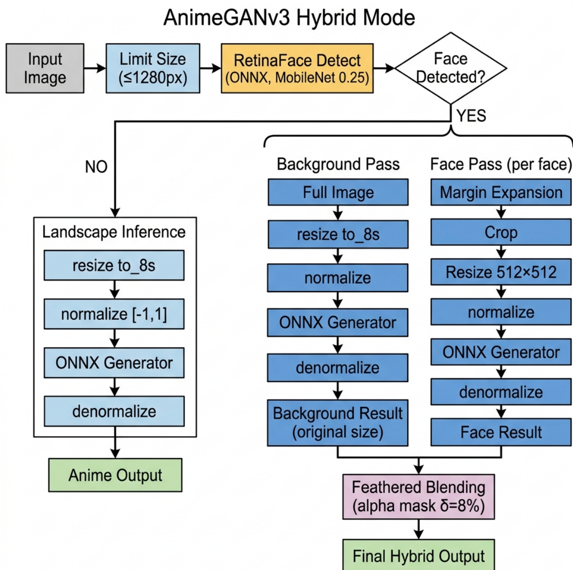
Hình 3.1. Pipeline tích hợp Face Extraction vào AnimeGANv3
