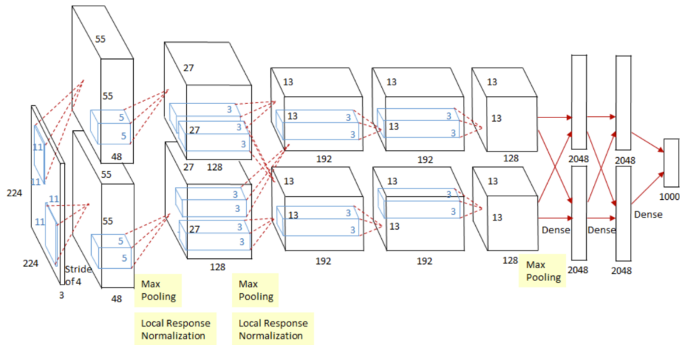
Hình 1.3. AlexNet
