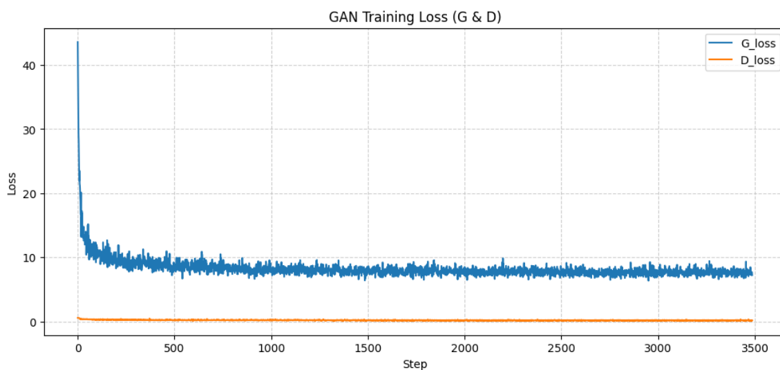
Hình 3.2. G_loss & D_loss
