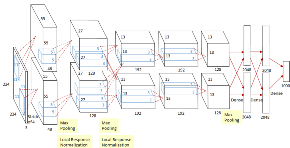
Hình 1.3. AlexNet
