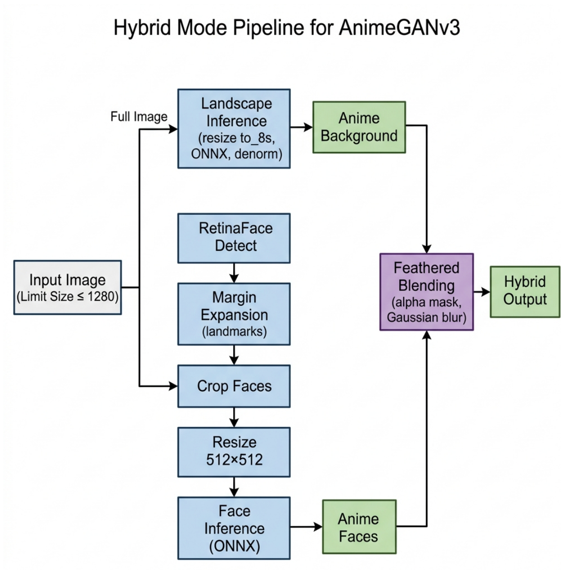
Hình 3.4. Pipeline xử lý Hybrid Mode: kết hợp Landscape Inference cho nền và Face Inference cho từng khuôn mặt
