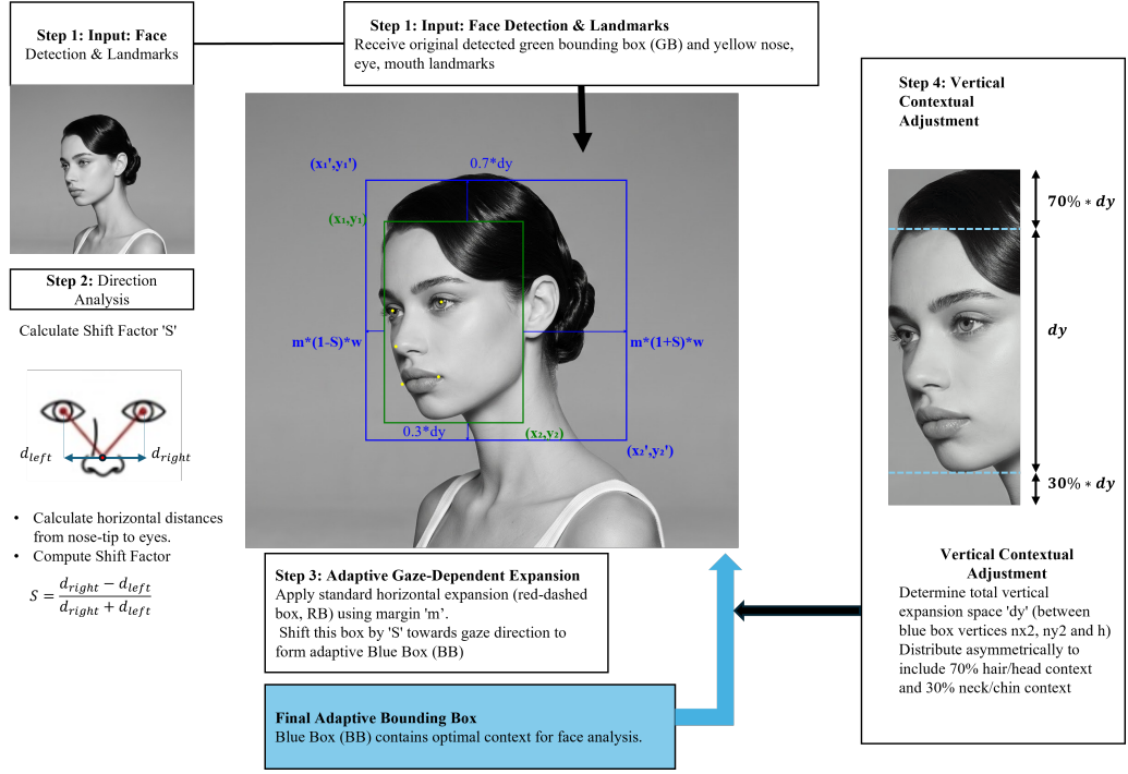
Hình 3.3. Minh họa kỹ thuật Margin Expansion
