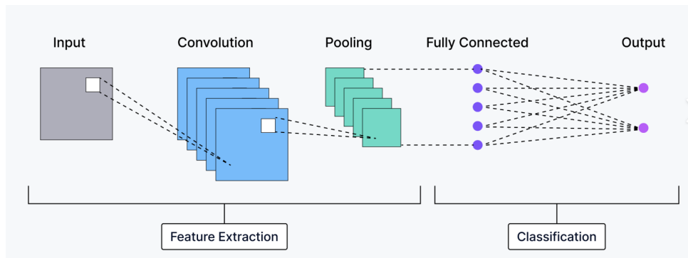
Hình 1.1. Kiến trúc cơ bản của Mạng Nơ-ron Tích chập
