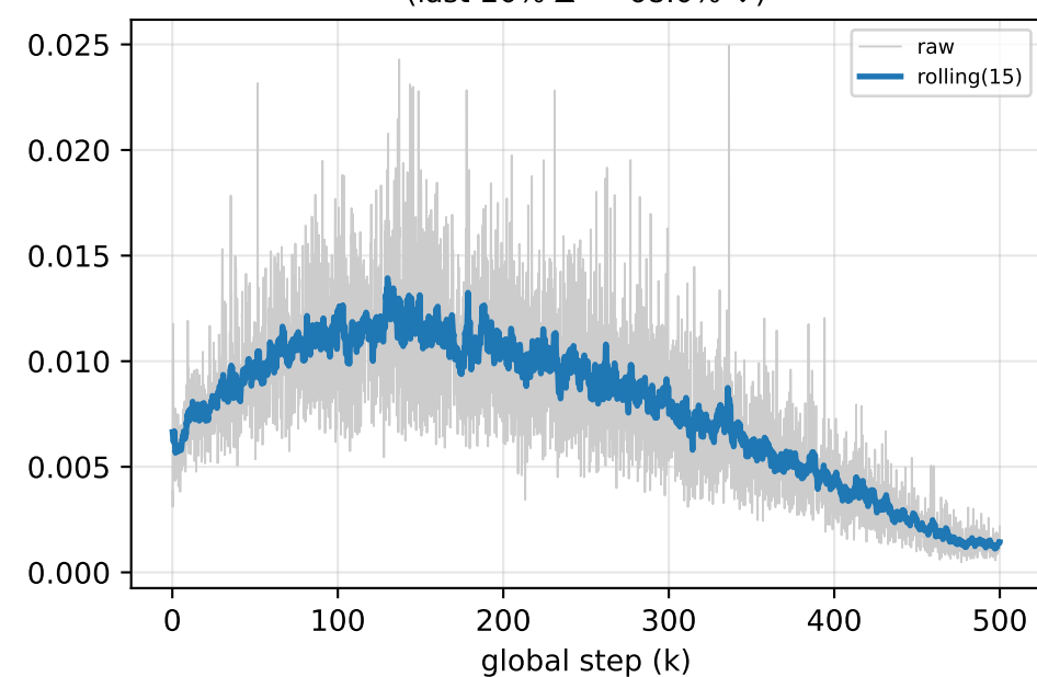
Approx KL (last-20% \Delta = -68.0\% \downarrow )
