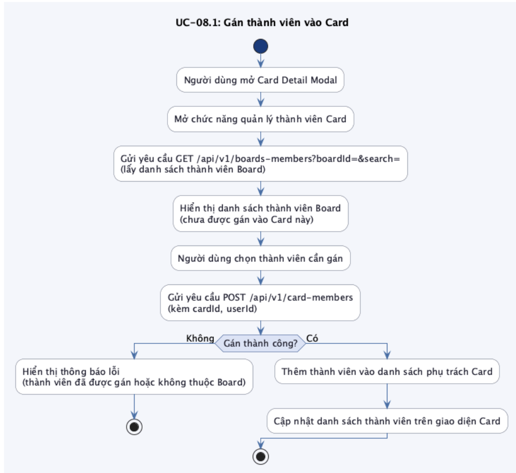
Hình 31: Biểu đồ hoạt động UC-08.1: Gán thành viên vào Card
