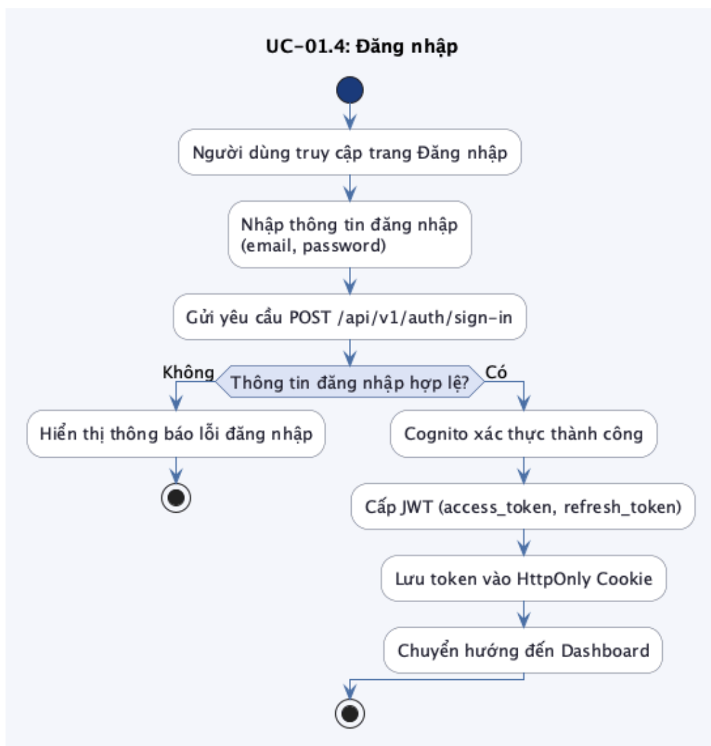
Hình 16: Biểu đồ hoạt động UC-01.4: Đăng nhập
