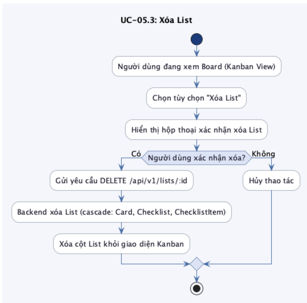
Hình 23: Biểu đồ hoạt động UC-05.3: Xóa List
