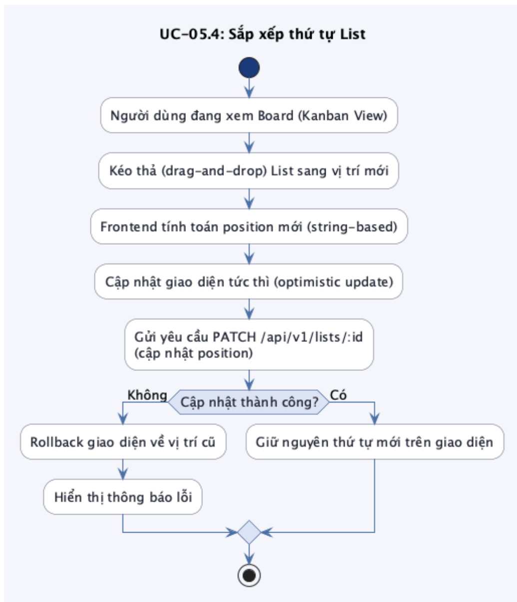
Hình 24: Biểu đồ hoạt động UC-05.4: Sắp xếp thứ tự List
