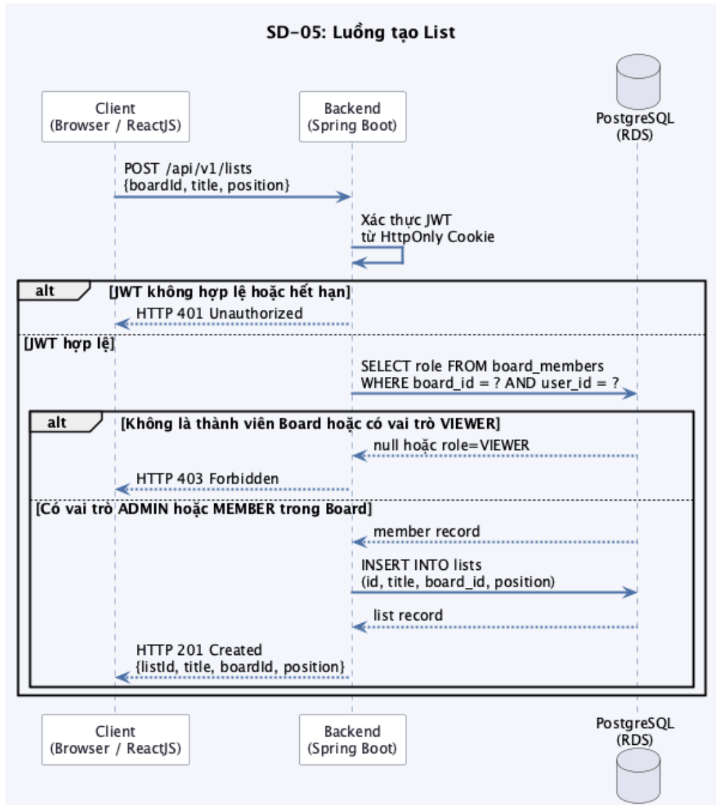
Hình 37: Biểu đồ tuần tự SD-05: Luồng tạo List
