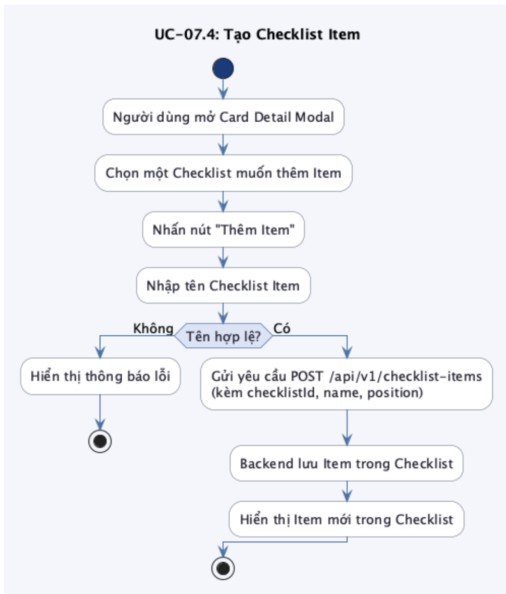
Hình 29: Biểu đồ hoạt động UC-07.4: Tạo Checklist Item
