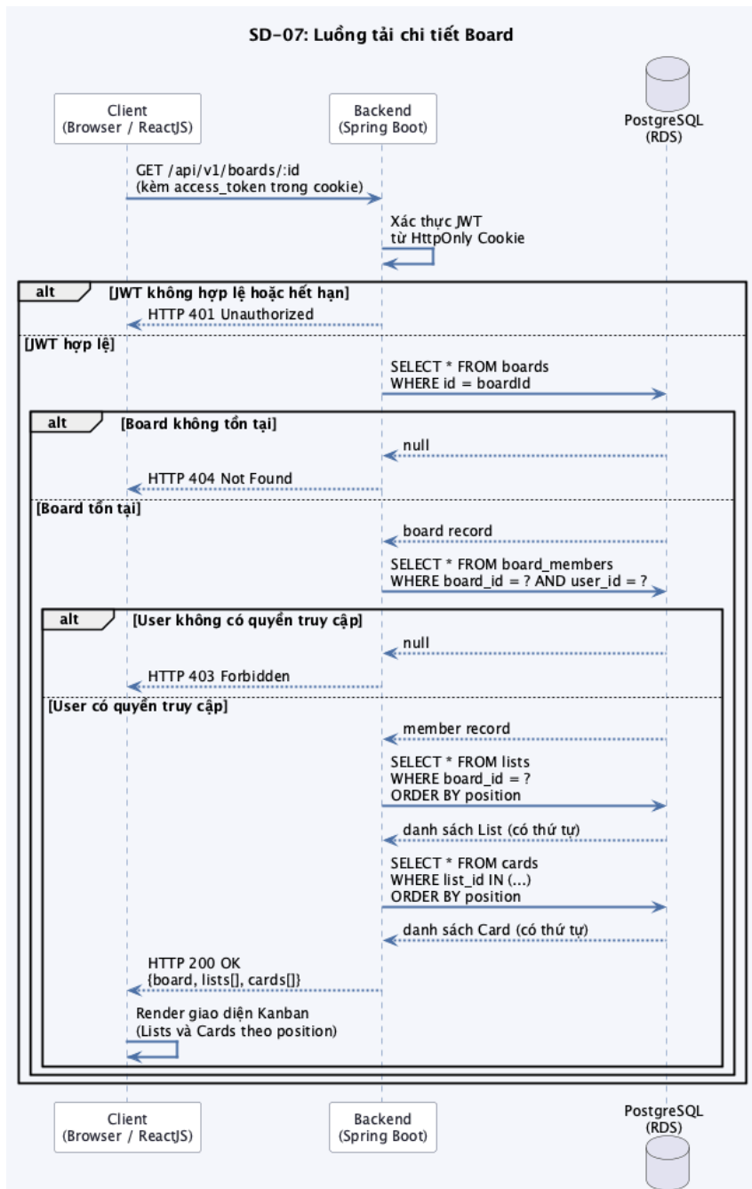
Hình 39: Biểu đồ tuần tự SD-07: Luồng tải chi tiết Board
