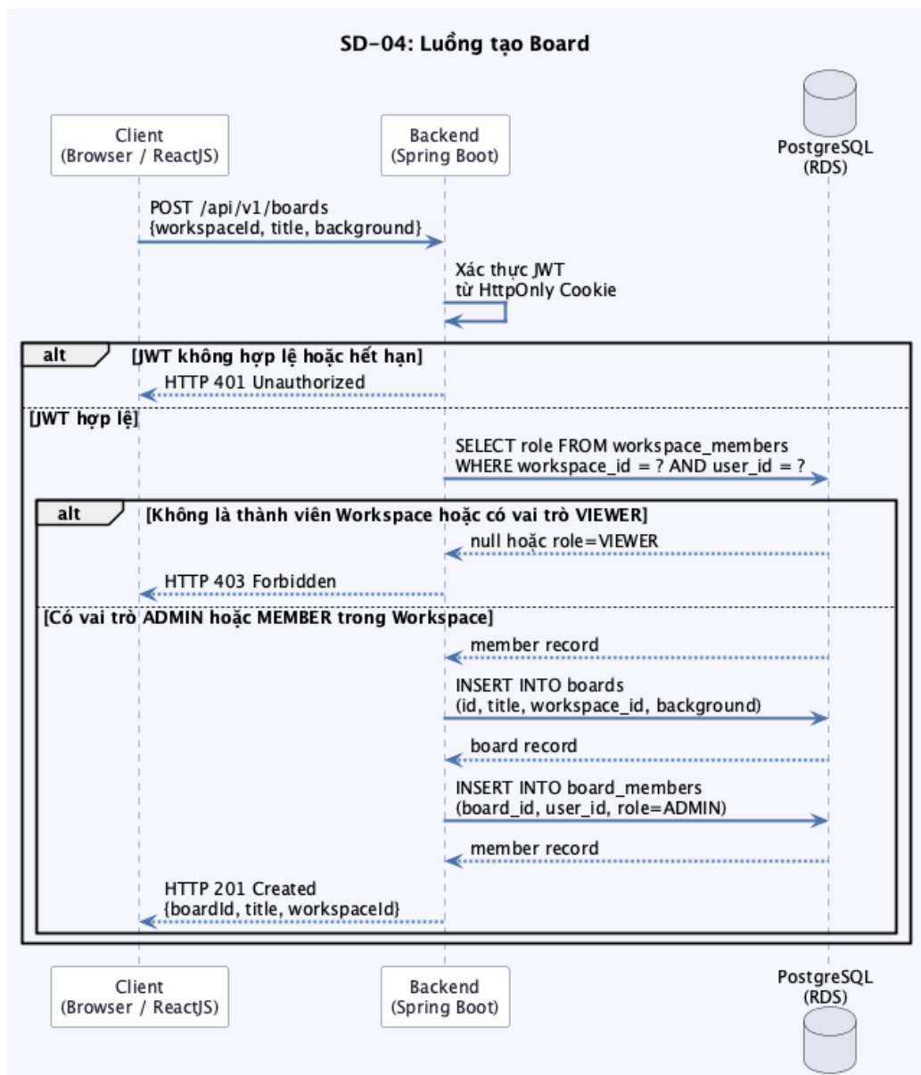
Hình 36: Biểu đồ tuần tự SD-04: Luồng tạo Board
