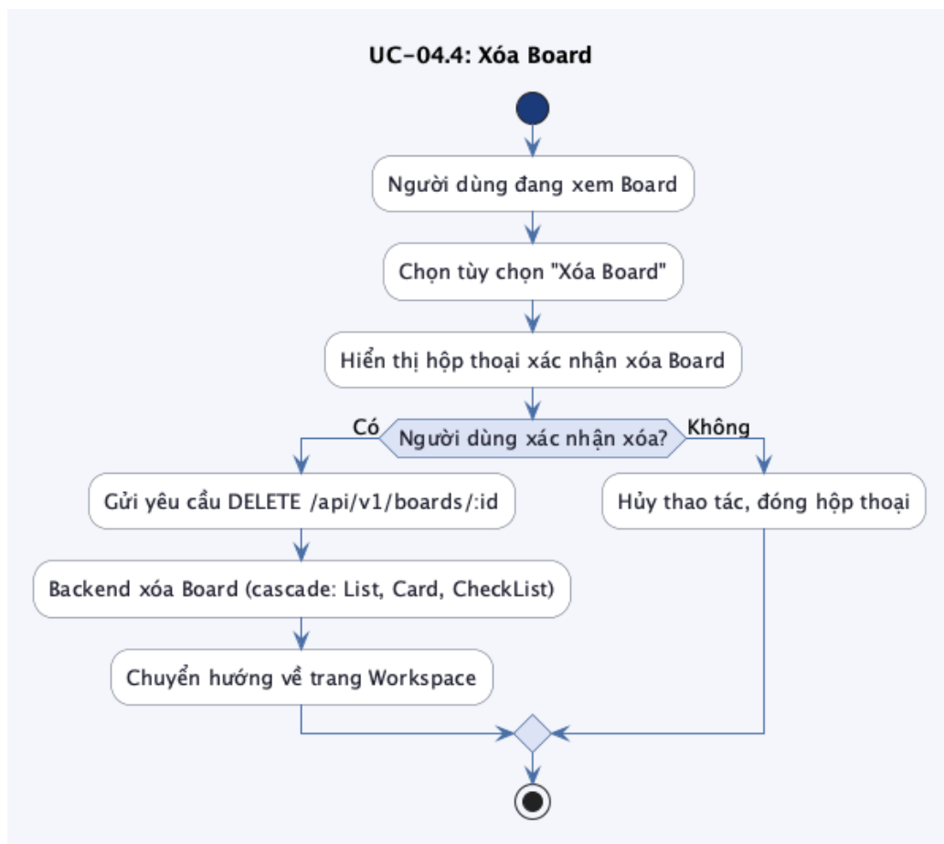
Hình 20: Biểu đồ hoạt động UC-04.4: Xóa Board
