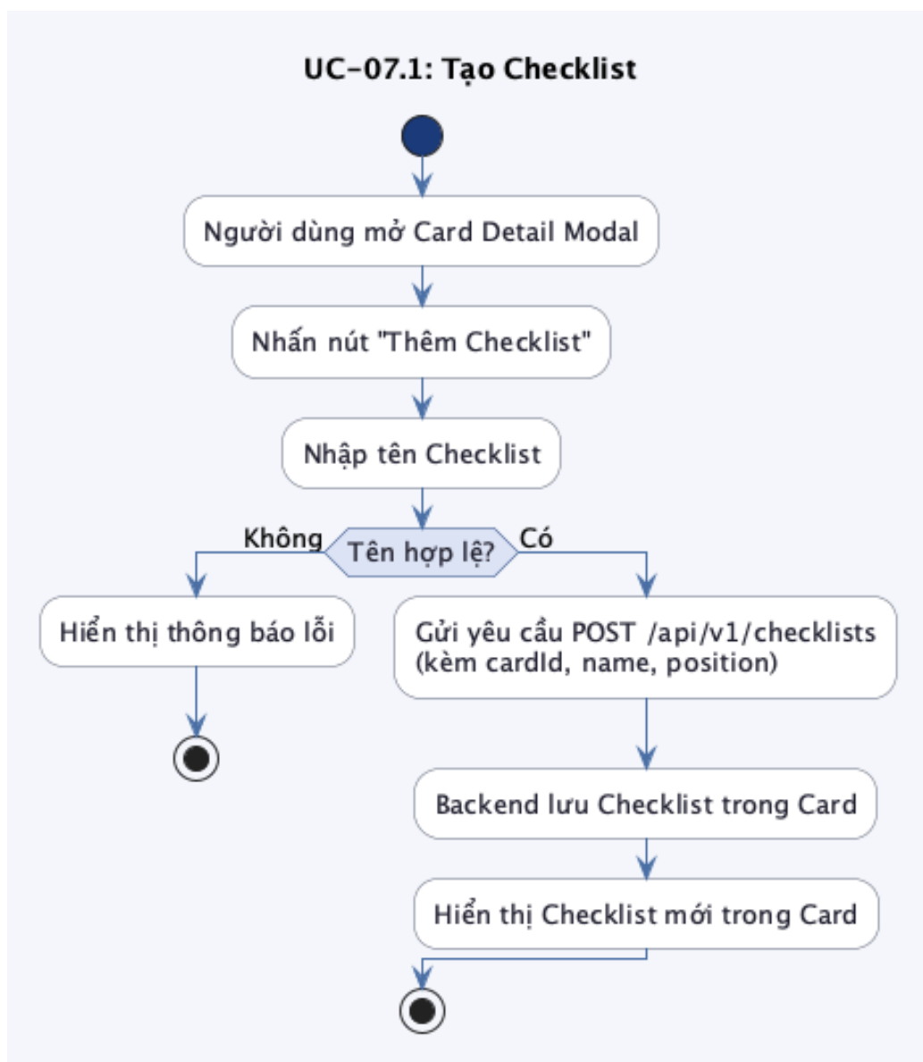
Hình 28: Biểu đồ hoạt động UC-07.1: Tạo Checklist
