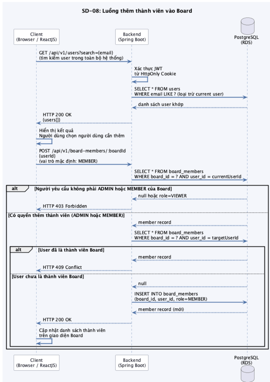
Hình 40: Biểu đồ tuần tự SD-08: Luồng thêm thành viên vào Board
