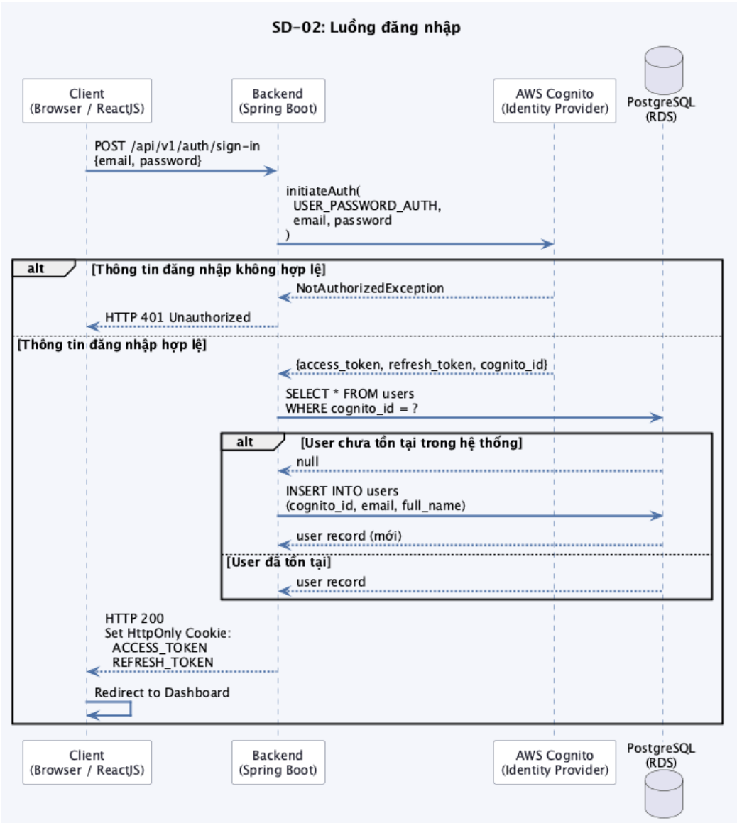
Hình 34: Biểu đồ tuần tự SD-02: Luồng đăng nhập
