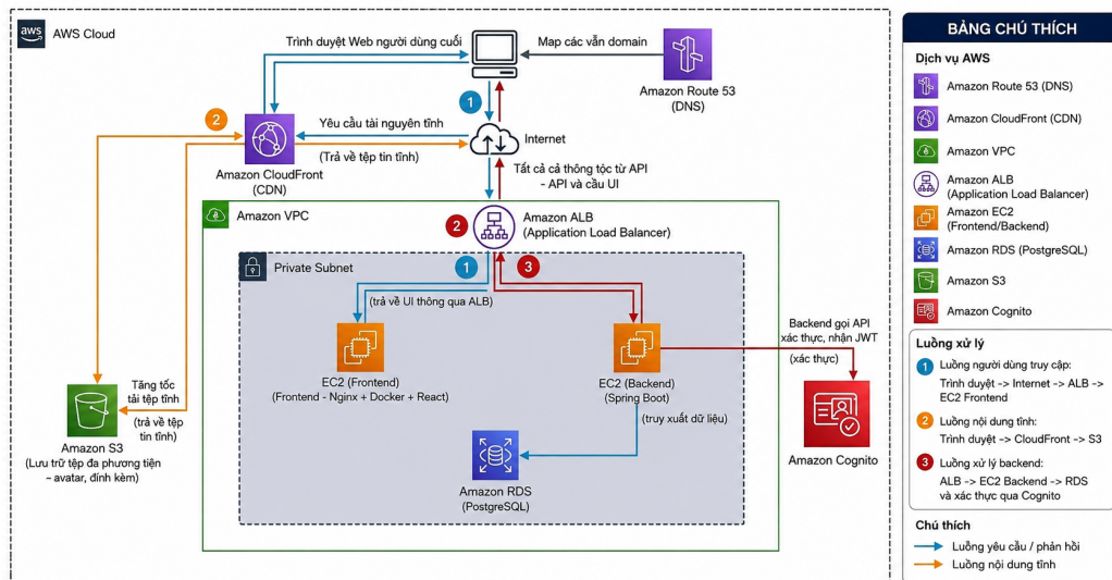
Hình 32: Kiến trúc triển khai hệ thống Nello trên AWS
