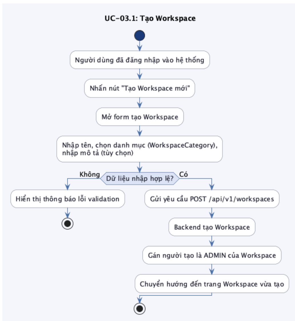
Hình 17: Biểu đồ hoạt động UC-03.1: Tạo Workspace
