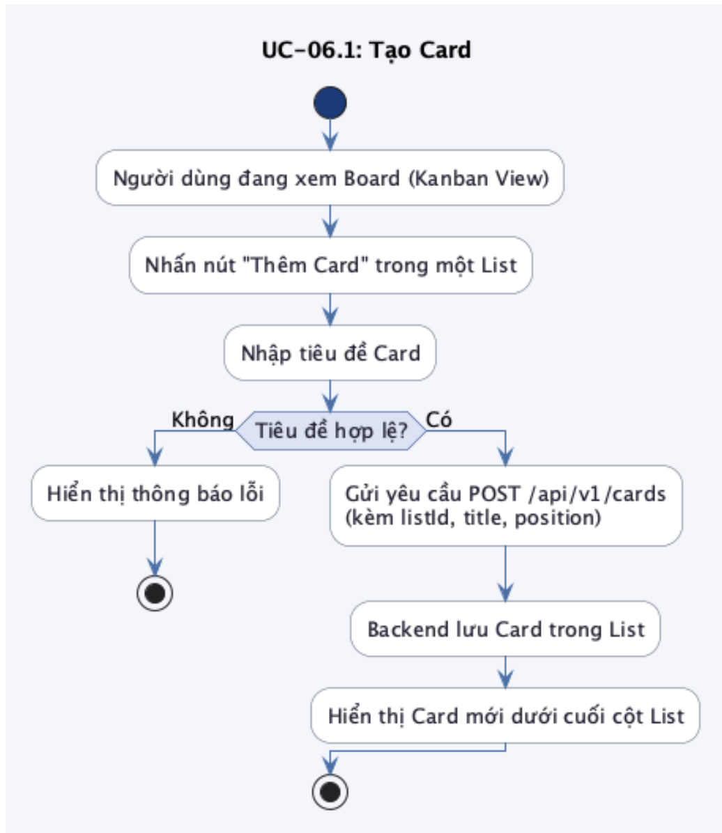
Hình 25: Biểu đồ hoạt động UC-06.1: Tạo Card
