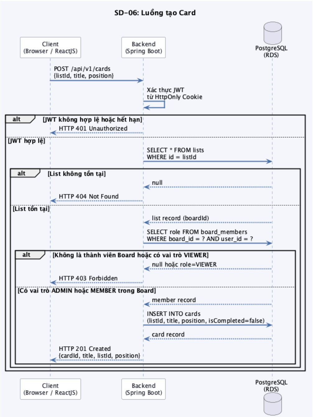
Hình 38: Biểu đồ tuần tự SD-06: Luồng tạo Card
