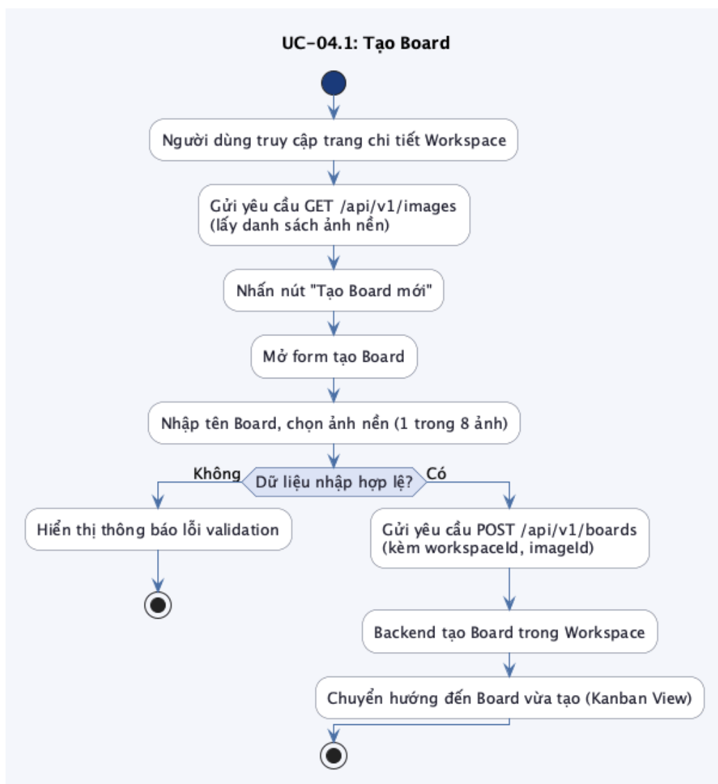
Hình 19: Biểu đồ hoạt động UC-04.1: Tạo Board
