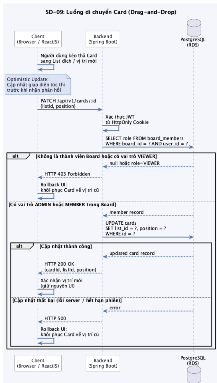
Hình 41: Biểu đồ tuần tự SD-09: Luồng di chuyển Card (Drag-and-Drop)
