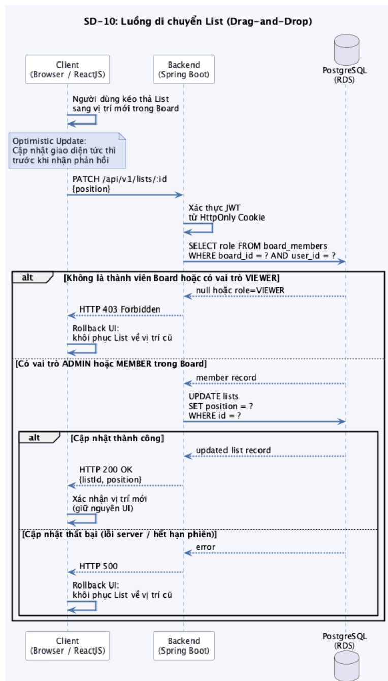
Hình 42: Biểu đồ tuần tự SD-10: Luồng di chuyển List (Drag-and-Drop)
