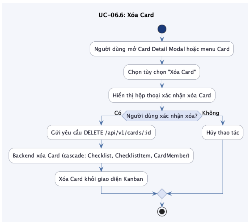
Hình 27: Biểu đồ hoạt động UC-06.6: Xóa Card
