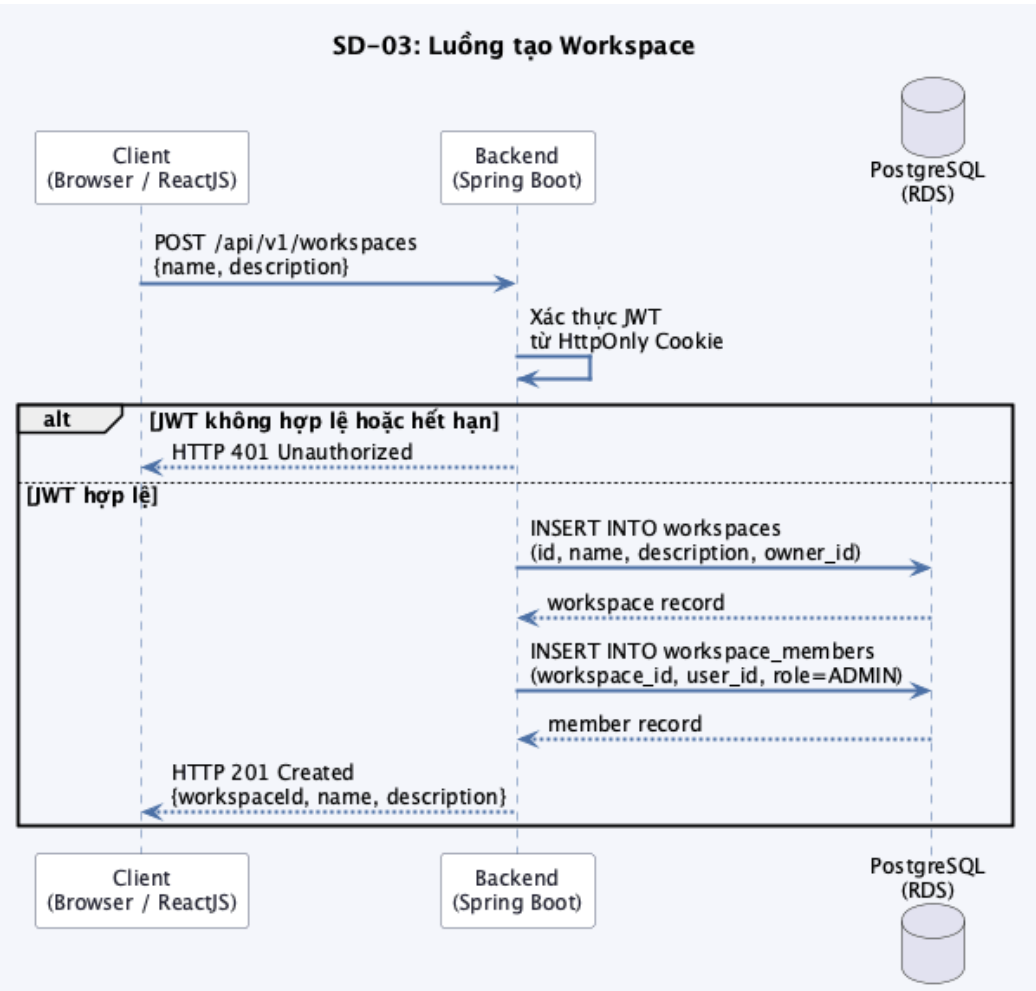
Hình 35: Biểu đồ tuần tự SD-03: Luồng tạo Workspace
