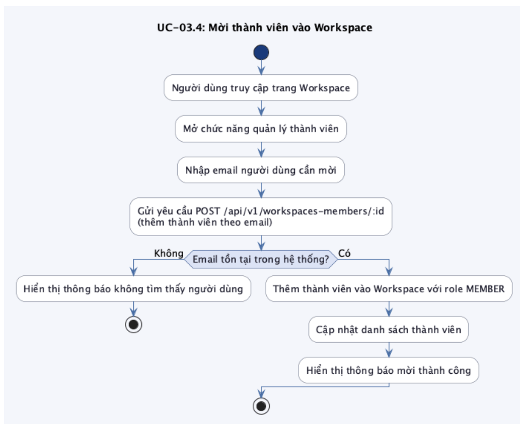
Hình 18: Biểu đồ hoạt động UC-03.4: Mời thành viên vào Workspace
