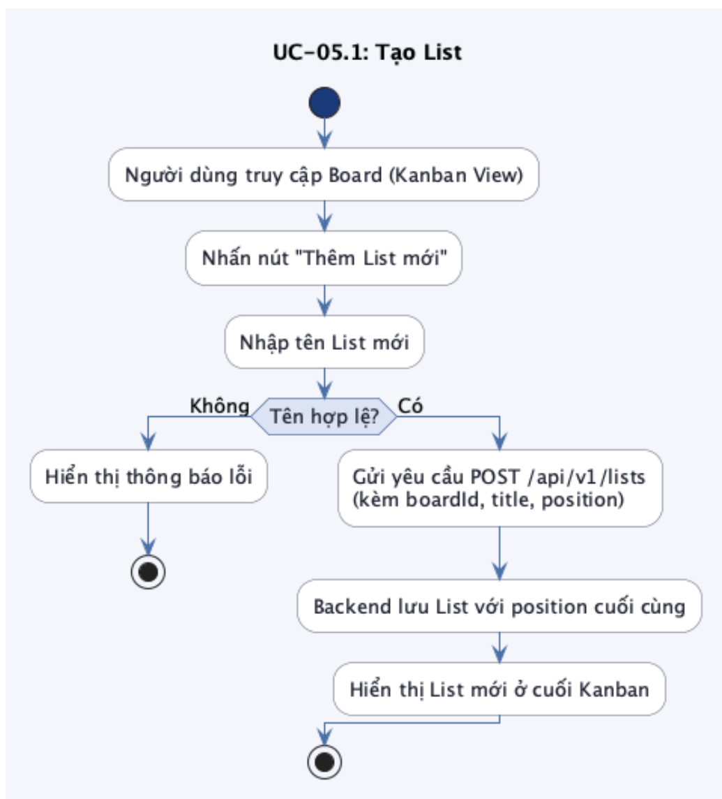
Hình 22: Biểu đồ hoạt động UC-05.1: Tạo List
