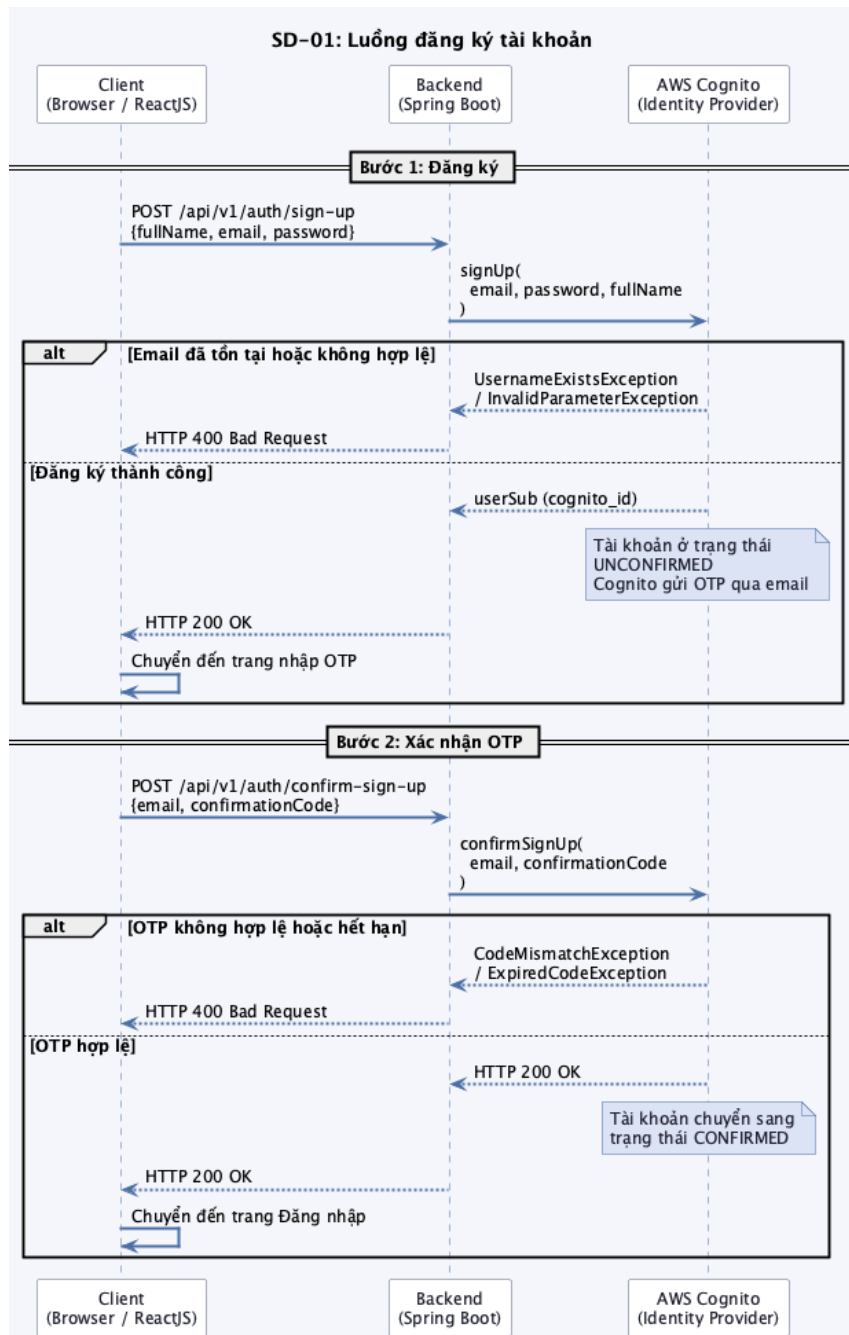
Hình 33: Biểu đồ tuần tự SD-01: Luồng đăng ký tài khoản
