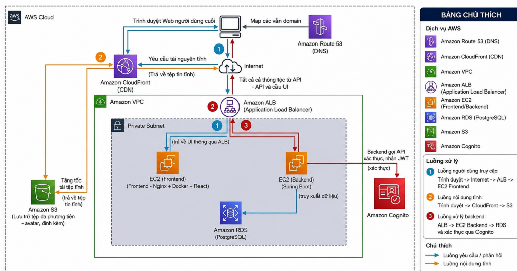
Hình 33: Kiến trúc triển khai hệ thống Nello trên AWS
