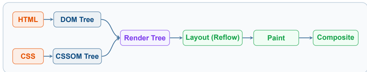
Hình 1.4: Cơ chế Critical Rendering Path của Trình duyệt Web
