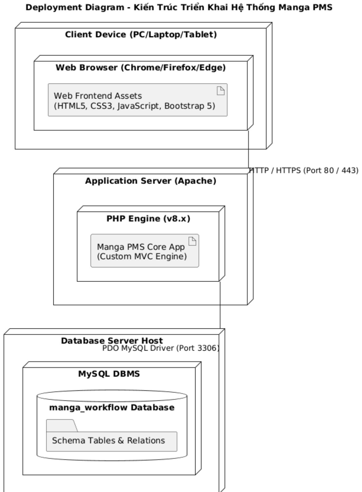
Hình IV.2: Kiến trúc triển khai hệ thống
