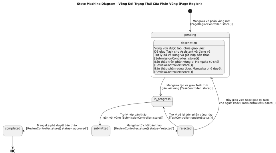
Hình IV.16: Biểu đồ trạng thái của Phân vùng trang truyện (PageRegion)
