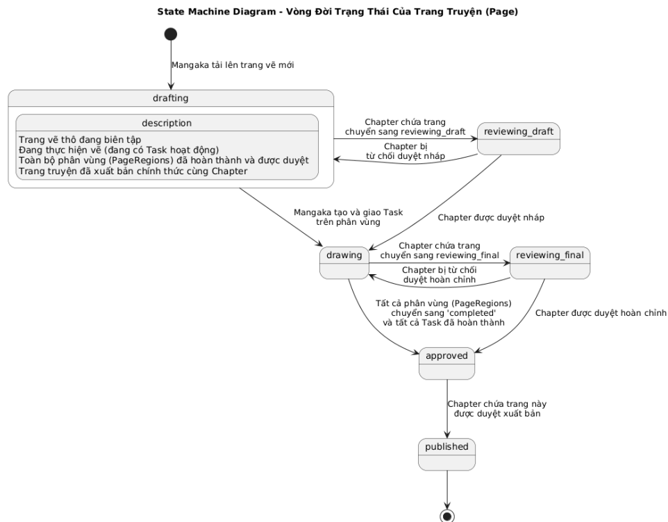
Hình IV.15: Biểu đồ trạng thái của Trang truyện (Page)
