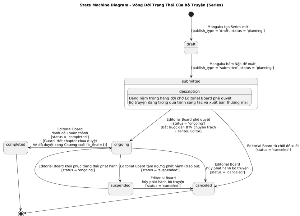
Hình IV.17: Biểu đồ trạng thái của Bộ truyện (Series)
