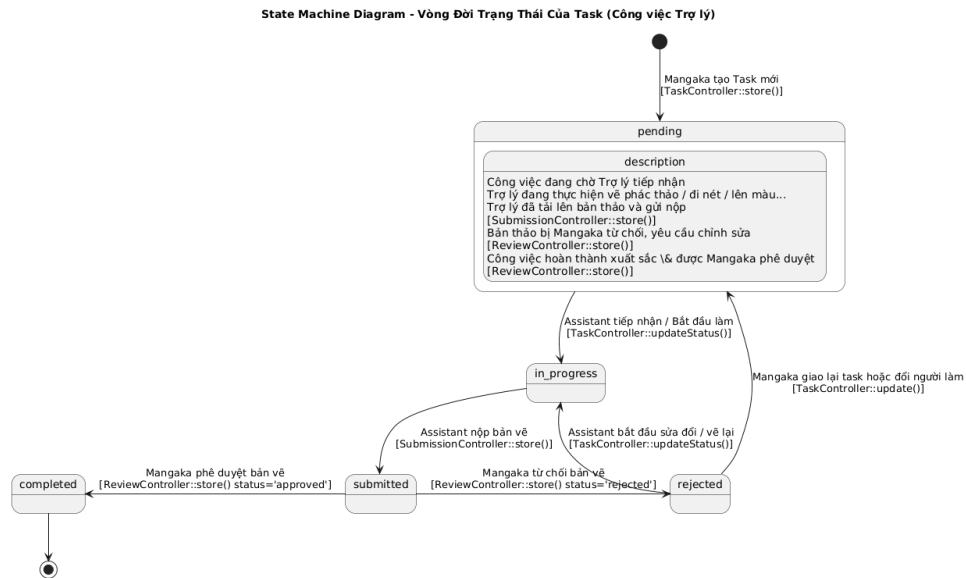
Hình IV.18: Biểu đồ trạng thái của Công việc (Task)
