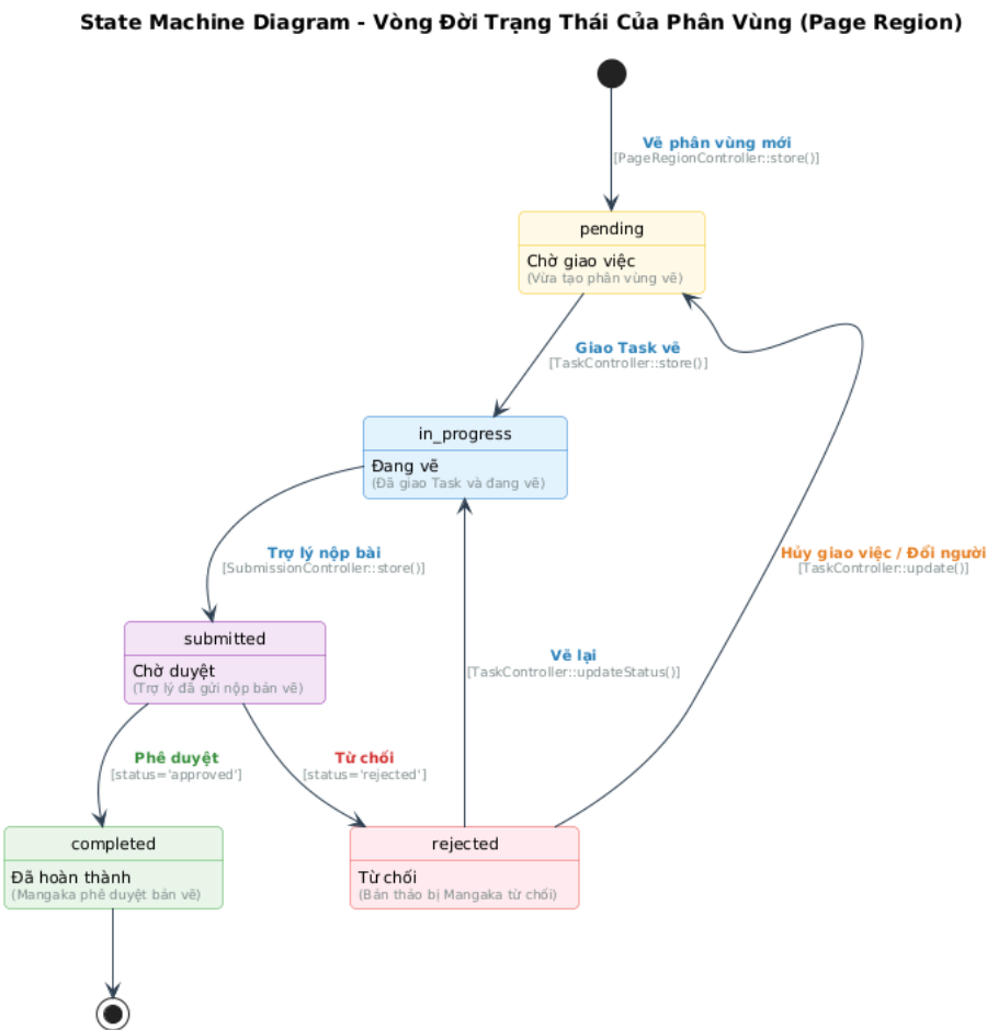
Hình IV.16: Biểu đồ trạng thái của Phân vùng trang truyện (PageRegion)
