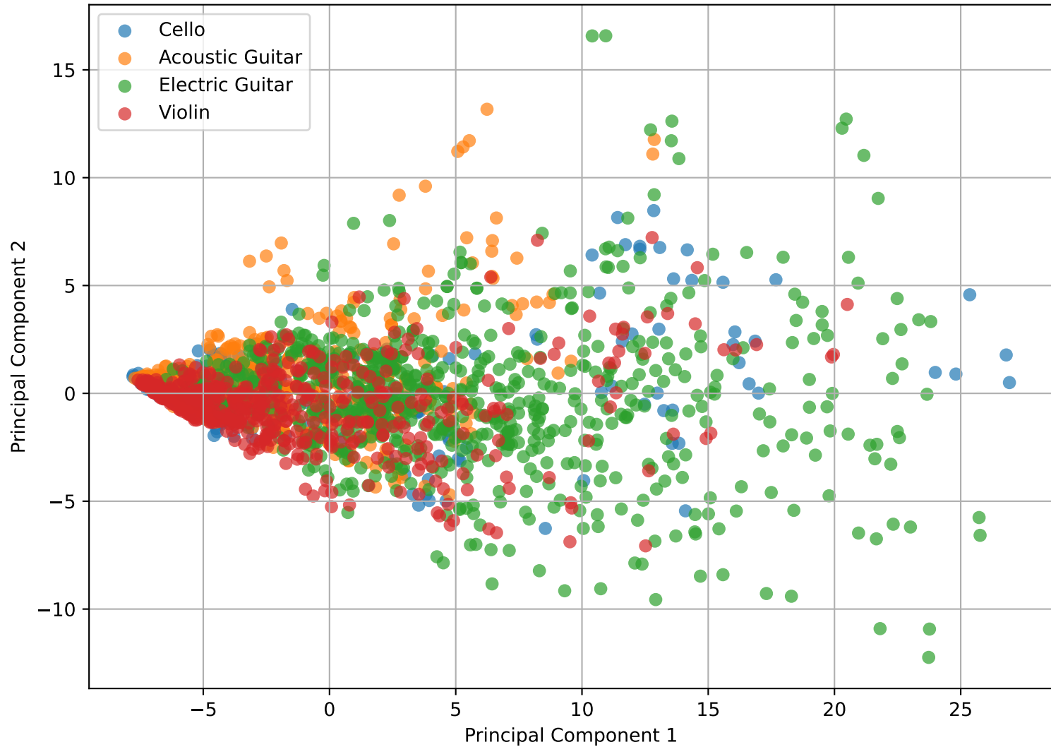
CQT PCA Visualization
