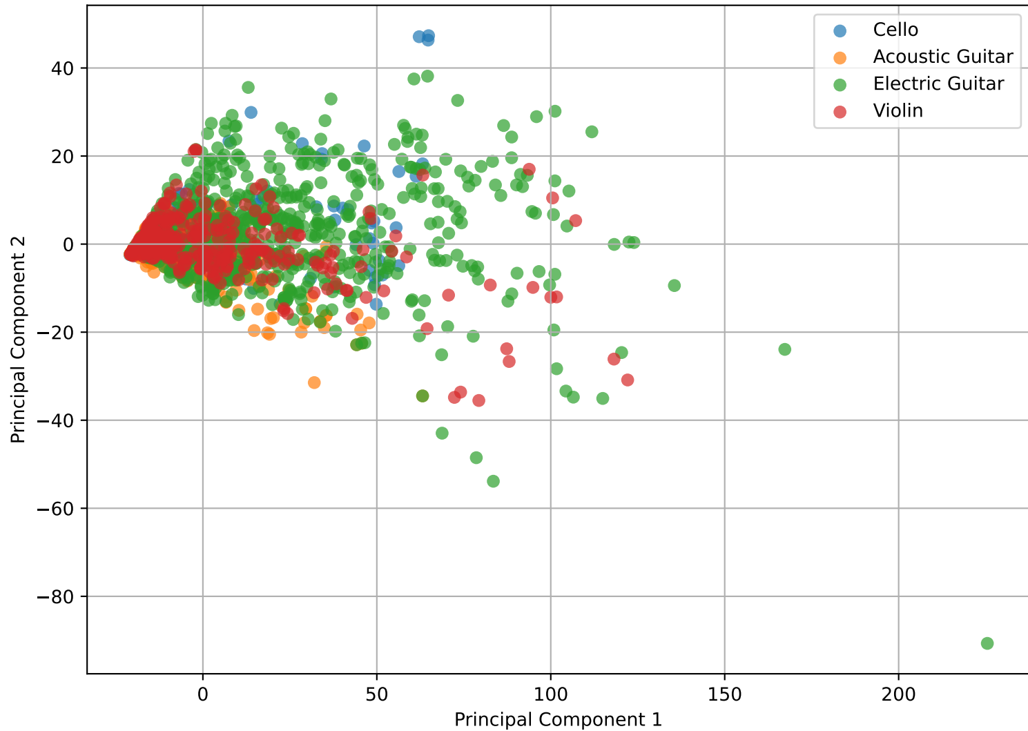
STFT PCA Visualization
