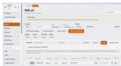
Hình 2b: Admin Portal — Quản Lý Kho & AI Generator: Kho 3.240 biển số, sinh prompt AI hàng loạt & sửa giá inline
