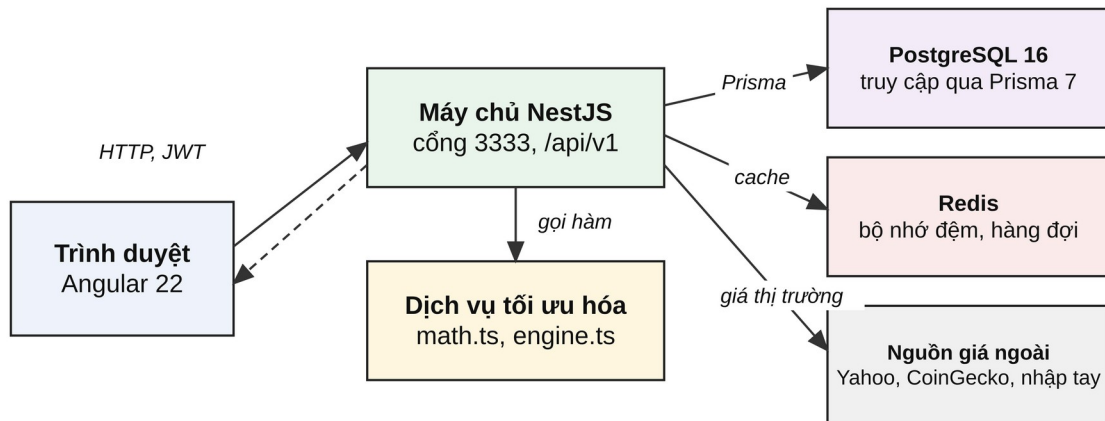
Hình 5.1. Kiến trúc hệ thống BL Advisor.
