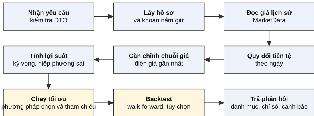
Hình 5.3. Luồng xử lý một yêu cầu tối ưu hóa, đọc từ trái sang phải ở hàng đầu rồi quay lại ở hàng sau.
