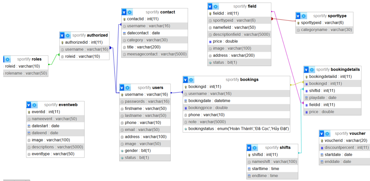
Hình 2. Lược đồ ERD
