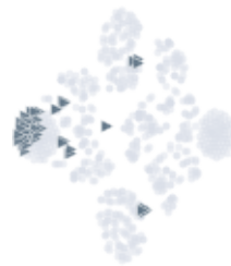
Claude Sonnet 5
