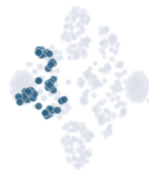
GPT-5 nano
