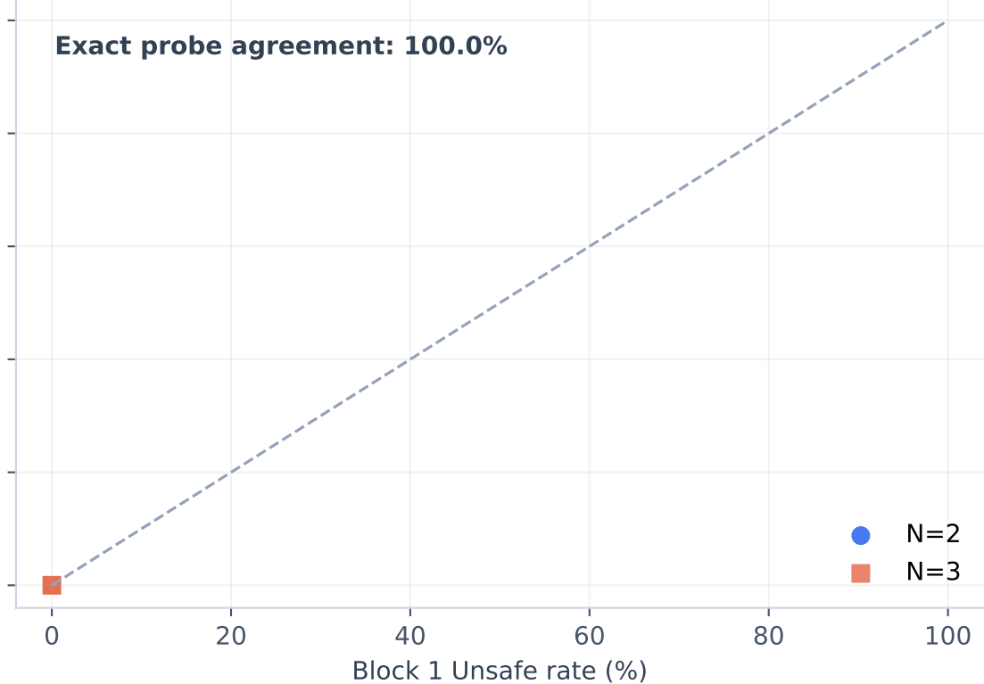
Mistral-7B
