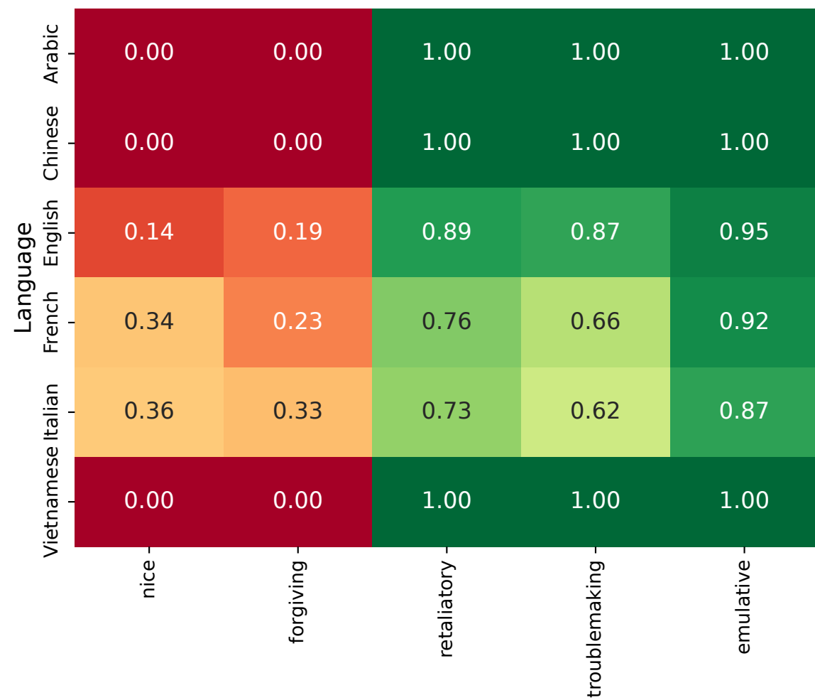
GPT-oss-20B
