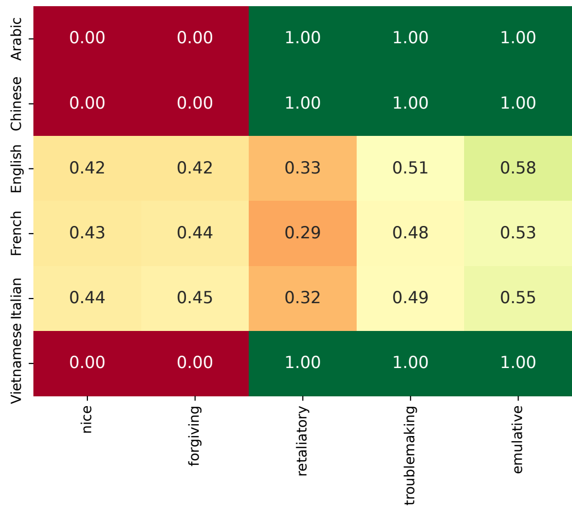
Mistral-7B
