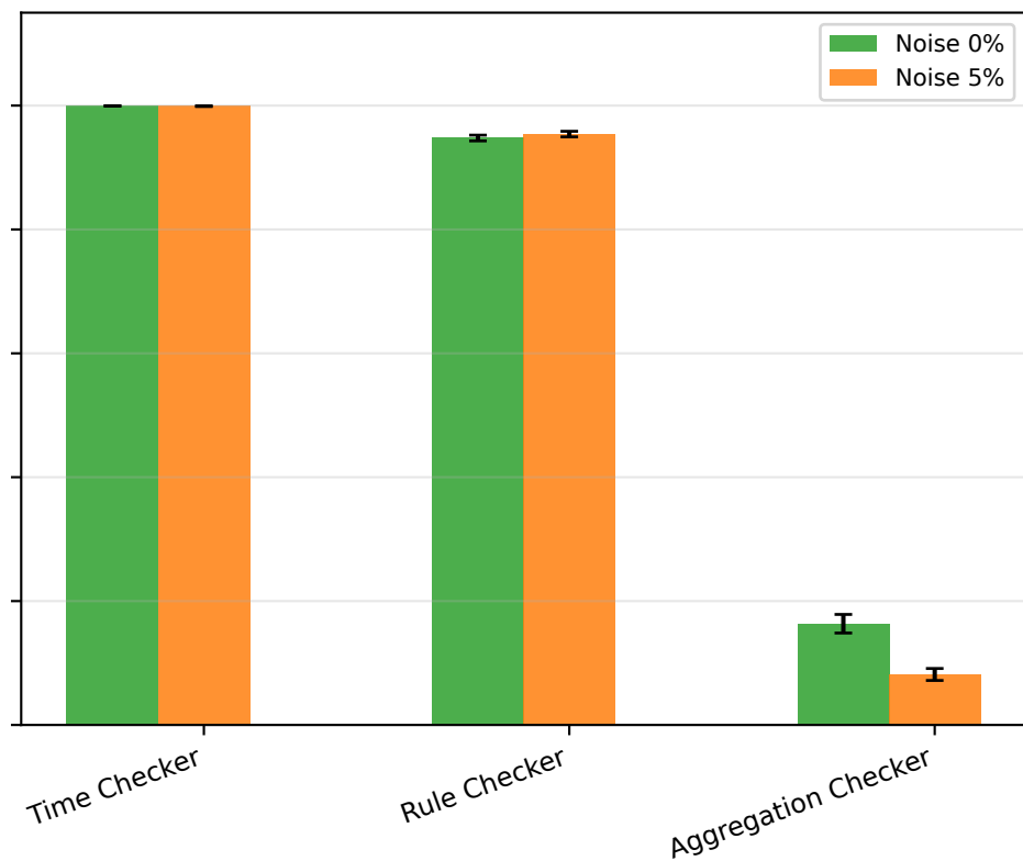
GPT-oss-20B
