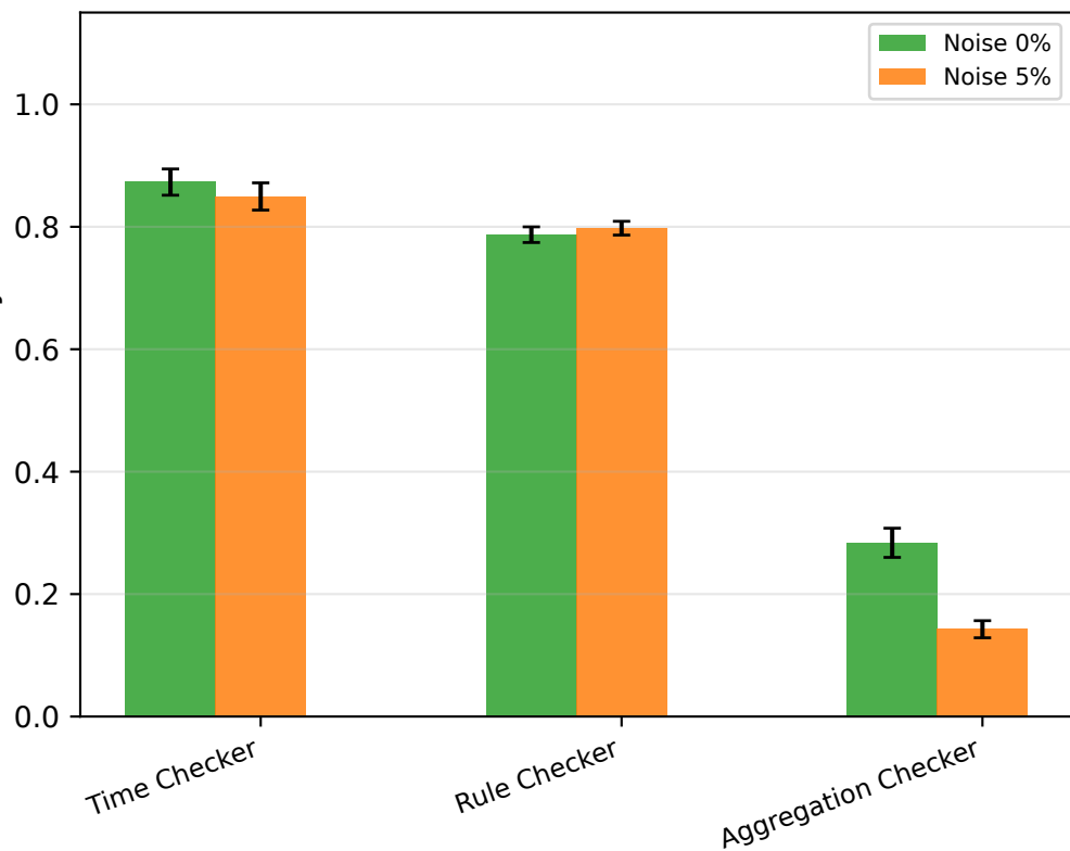
Mistral-7B
