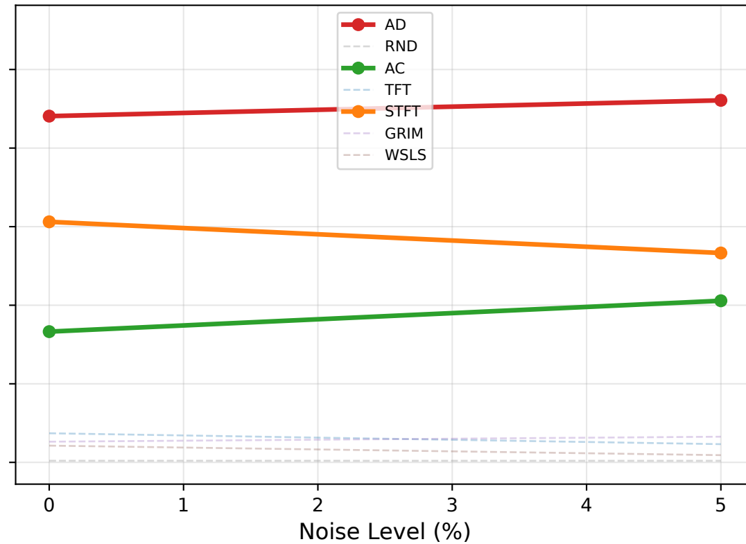
Mistral-7B
