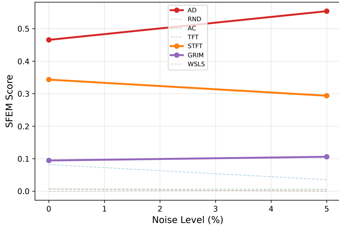
GPT-oss-20B
