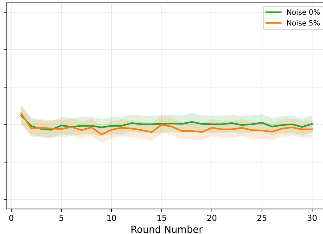
Mistral-7B
