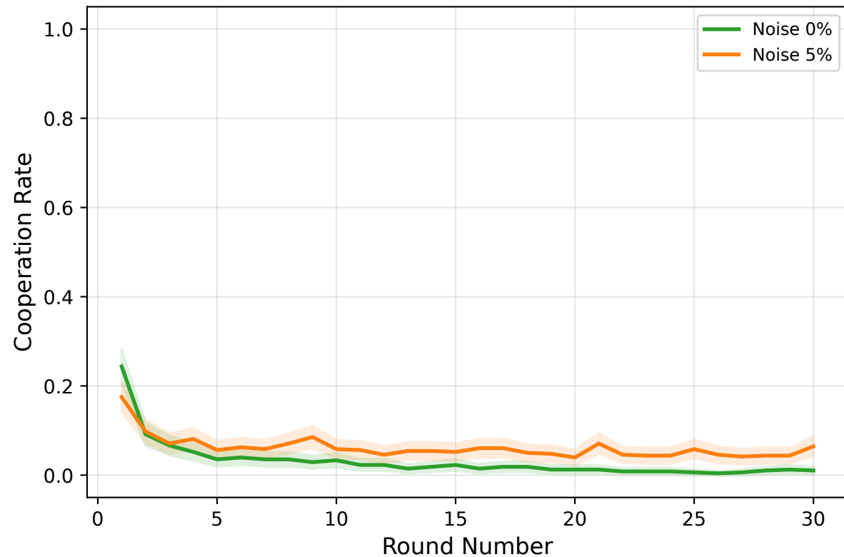
GPT-oss-20B
