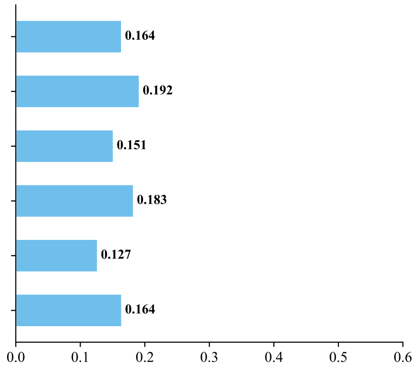
Mistral-7B
