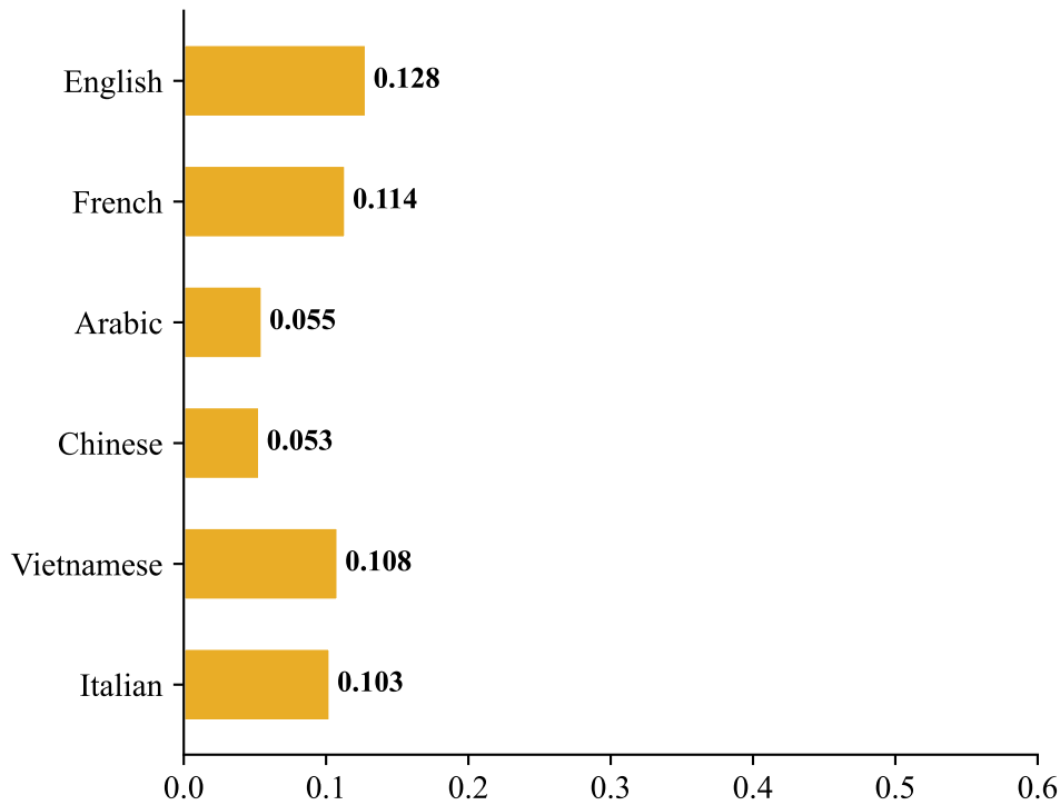
GPT-oss-20B
