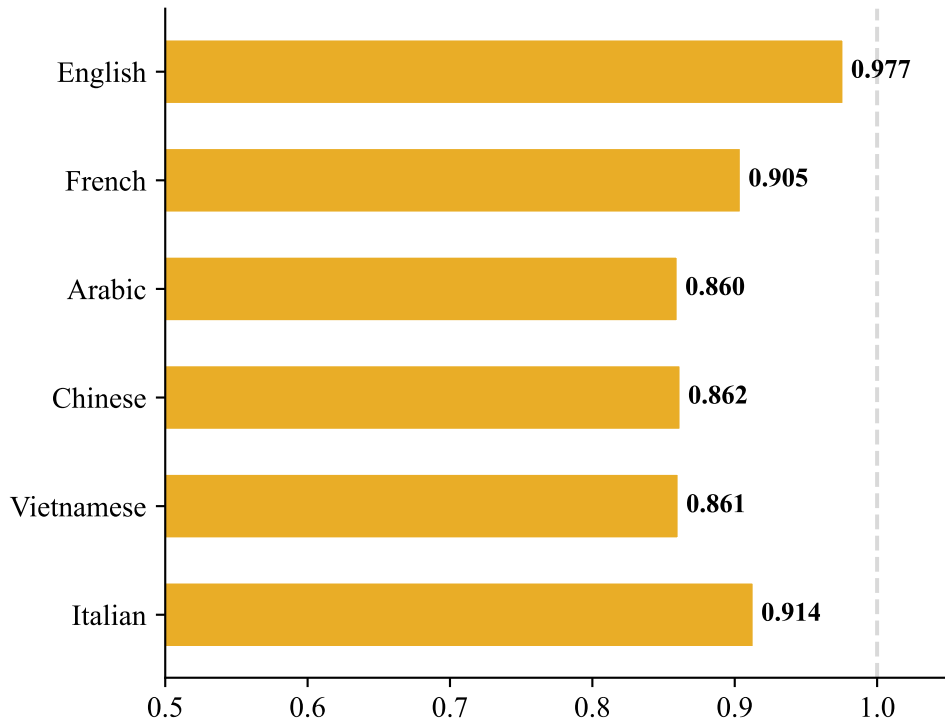
GPT-oss-20B
