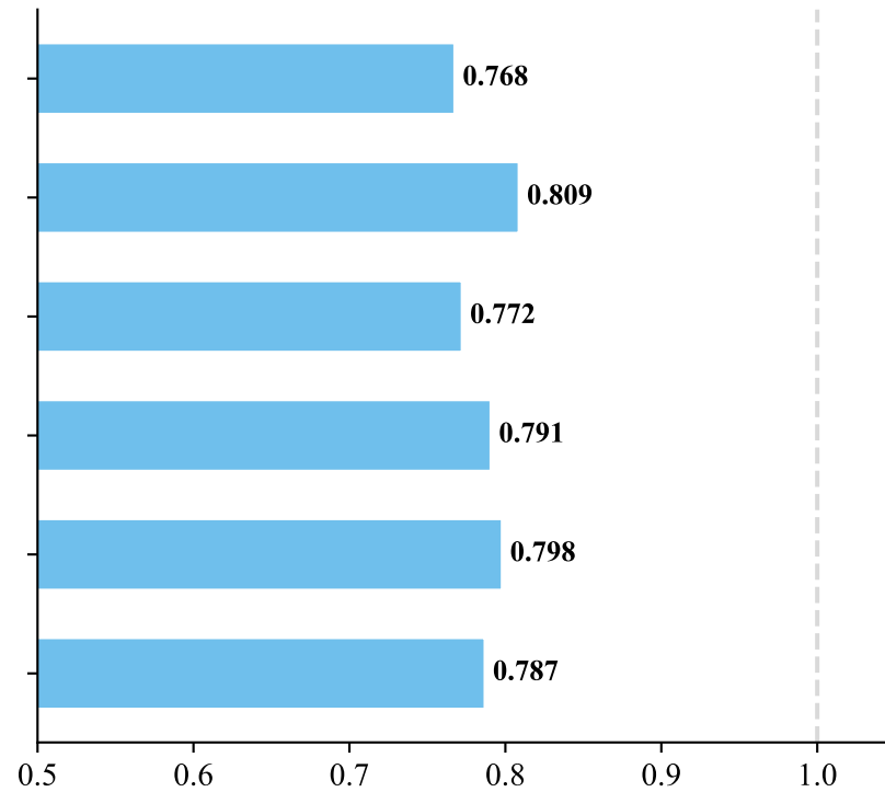
Mistral-7B
