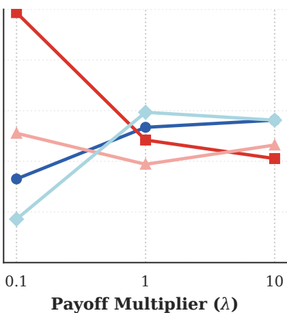
GPT-4o
