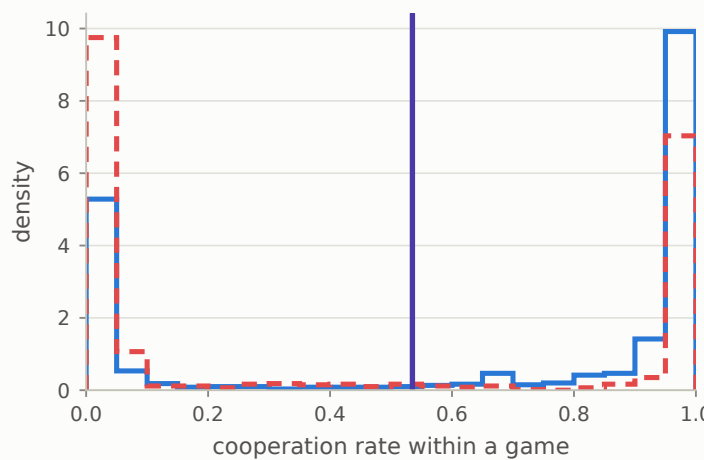
Gemma-3-12B
