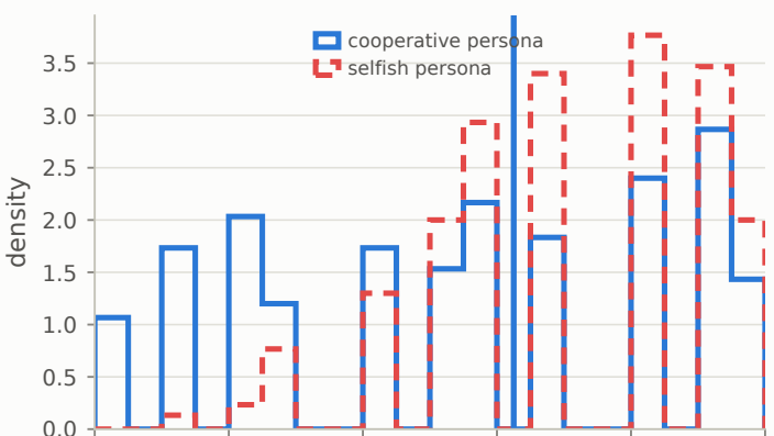
Gemma-3-12B
