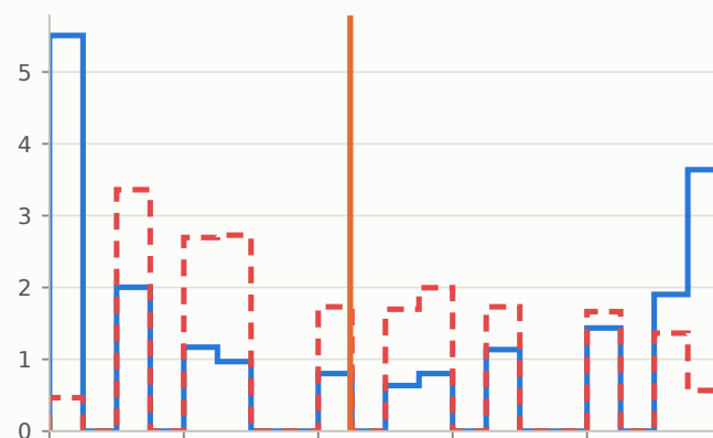
Llama-3.1-8B
