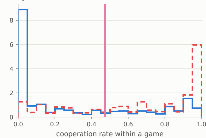
Qwen3-8B
