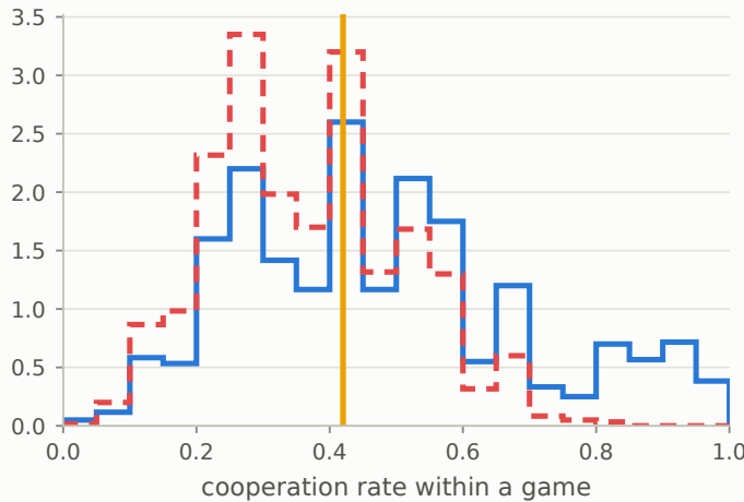
Llama-3.1-8B
