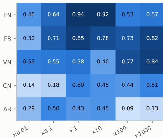
Gemma-3-12B
