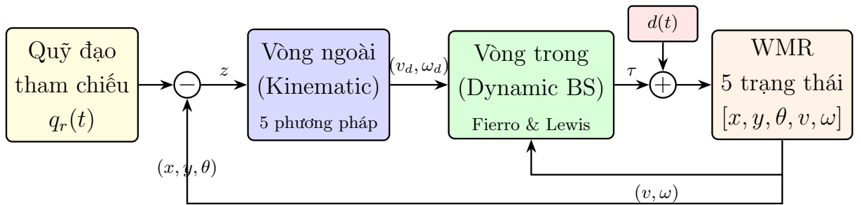
Figure 4.1: Kiến trúc điều khiển hai vòng: vòng ngoài tính vận tốc mong muốn (v_d, \omega_d) , vòng trong chuyển thành mô-men \tau , nhiễu d(t) tác động trực tiếp vào mô-men
