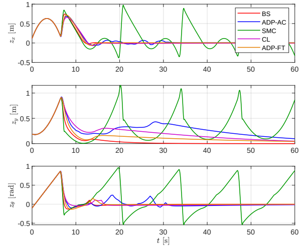
Figure 4: Sai số bám đường tròn.
