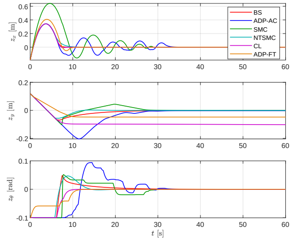
Figure 5.4: Sai số z(t) – Đường thẳng
