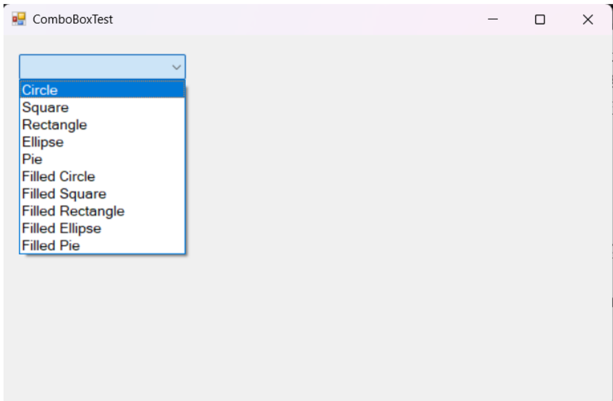
Hình 4-2 GUI Bài 09 - 1
