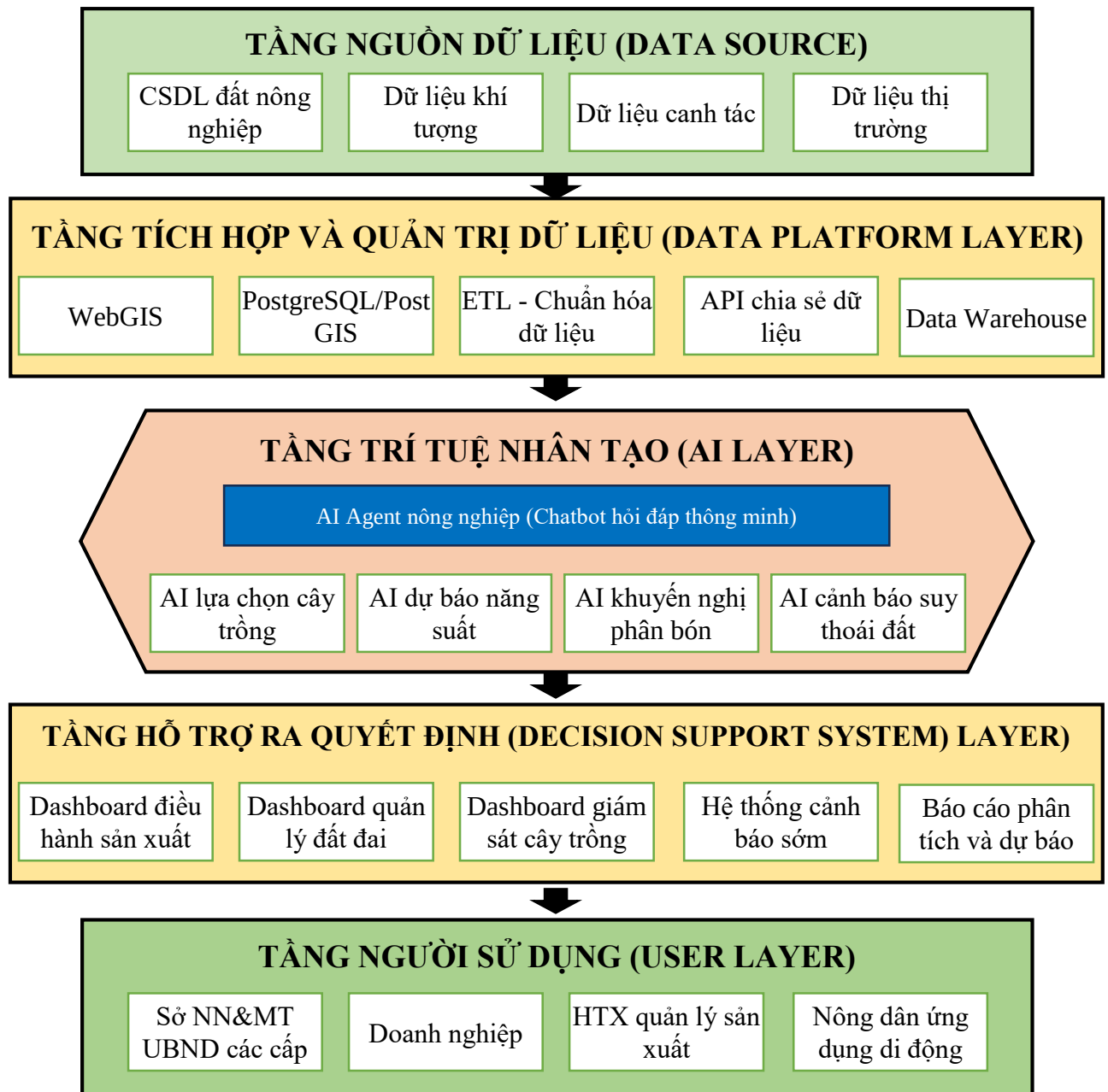
Hình 7. Kiến trúc hệ thống AI khai thác cơ sở dữ liệu
