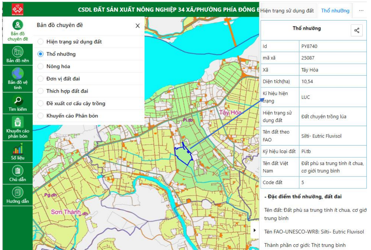
Hình 3. Cơ sở dữ liệu không gian và thuộc tính về thổ nhưỡng.
