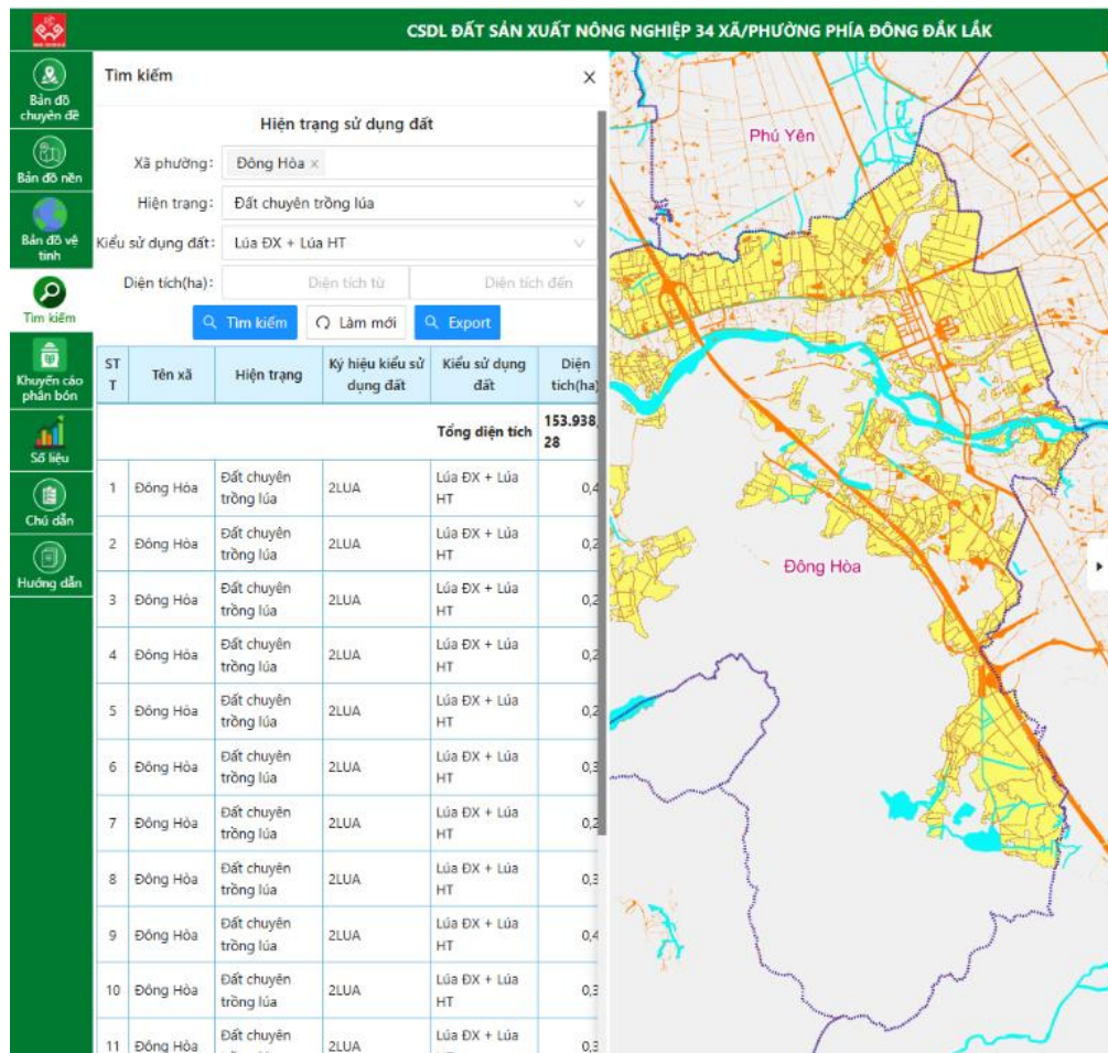
Hình 5. Chức năng tìm kiếm trên cơ sở dữ liệu WebGIS.
