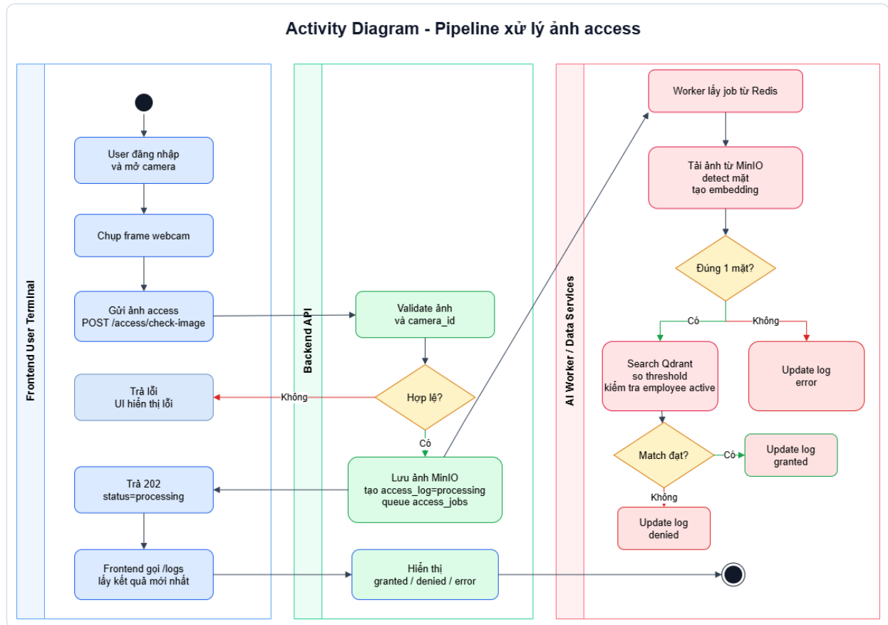
Hình 1.2: Activity diagram cho pipeline xử lý ảnh access
