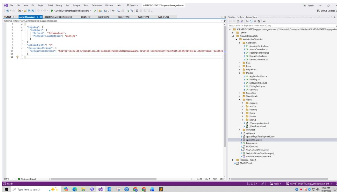
Hình 7: Sơ đồ cấu trúc thư mục theo mô hình MVC
