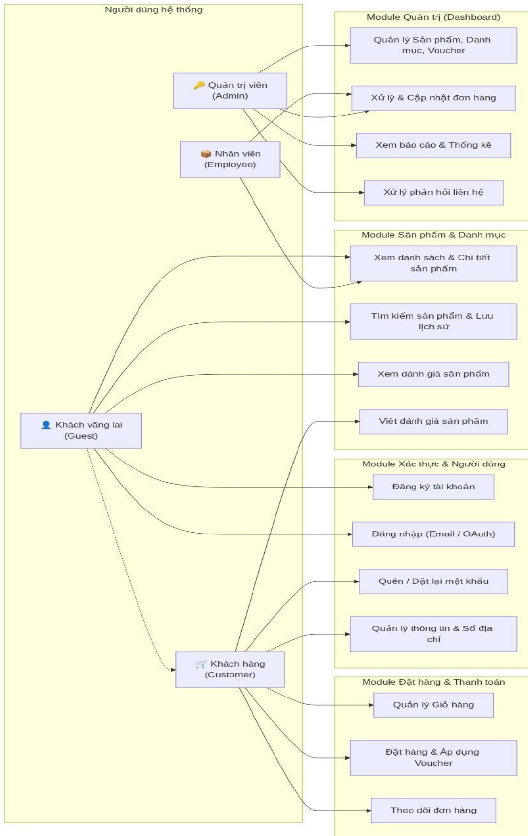
Hình 1. Kiến trúc tổng thể hệ thống TechVie
