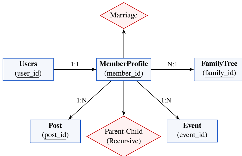
Hình 2.1: Sơ đồ các mối liên kết cốt lõi của hệ thống FamilyConnect (Graph Data Model).
