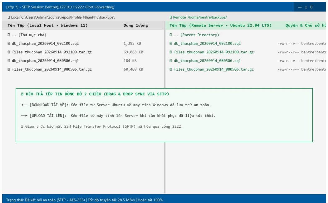
Hình 4.10: Giao diện màn hình truyền tệp SFTP đồ họa 2 chiều Xftp giữa máy thật và máy ảo
