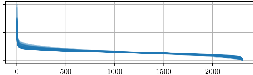
Layer 18
