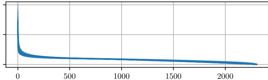
Layer 6
